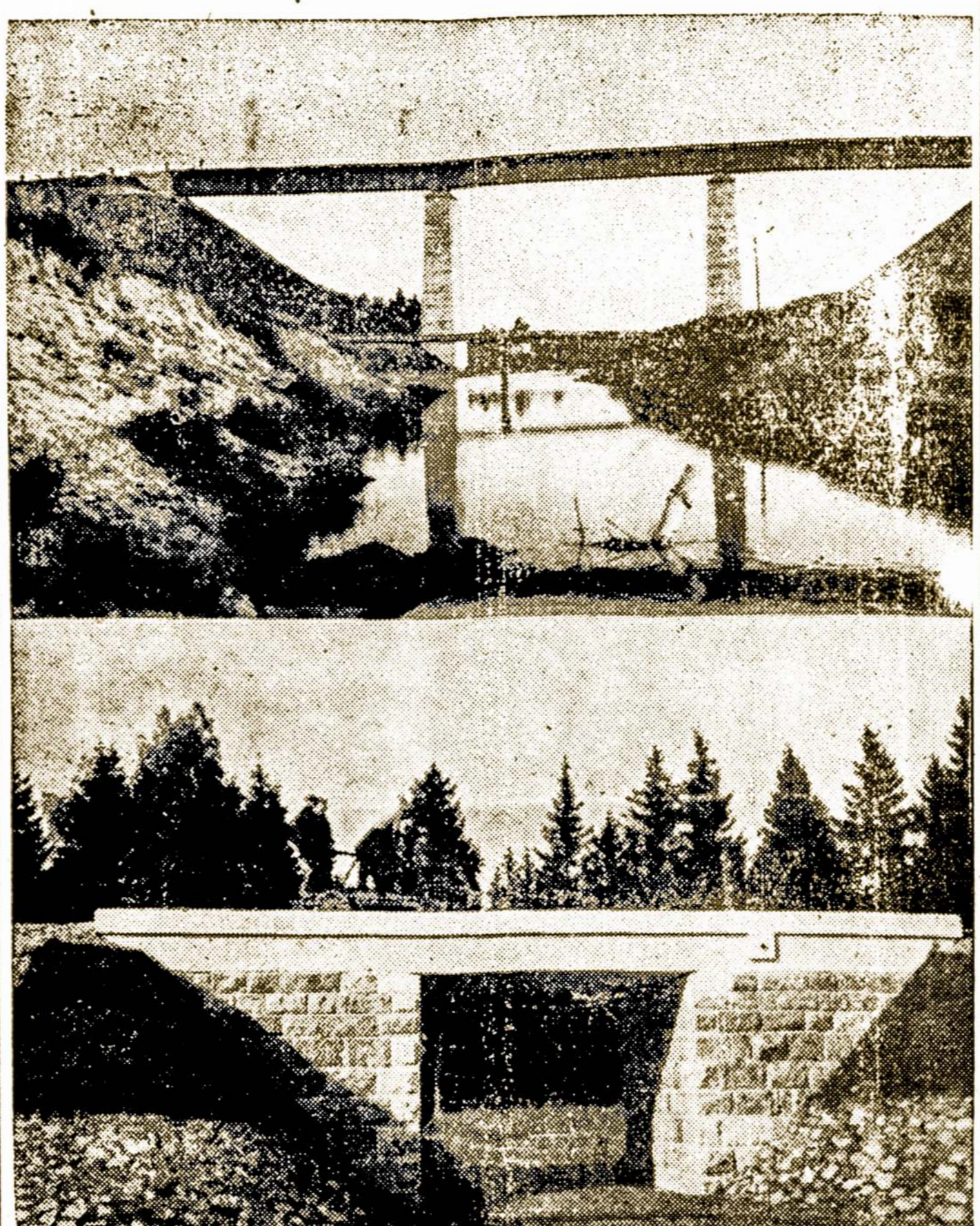
LIETUVOS PAZANGOS VAIZDAI Telšių — Kretingos geležinkelis, prieš keletą metų pastatytas jungia Didž. Lietuvą su Klaipėdos kraštu ir uostu. Šis geležinkelis gražiai pastatytas, ką rodo čia matomi jo tiltai.
