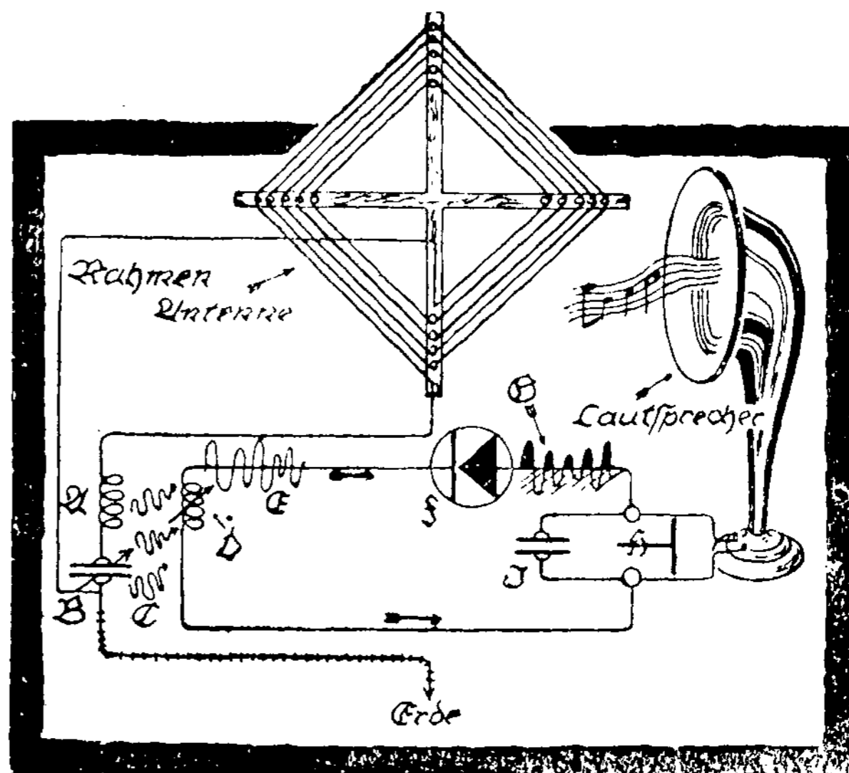
Paprasto detektorinio radioimtuvo skema. Paaiškinimai: Rahmen-Antenne = rėminė antena, Erde = žemė, Lautsprecher = garsiai kalbantis telefonas.
