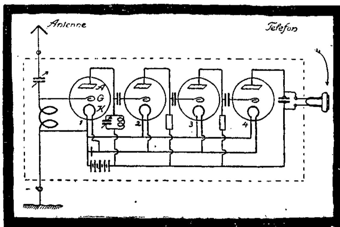
Katodinių vamzdelio radioimtovo skėma su 4 katodinais vamzdeliais. (Spiralgitter = tinklelis).
