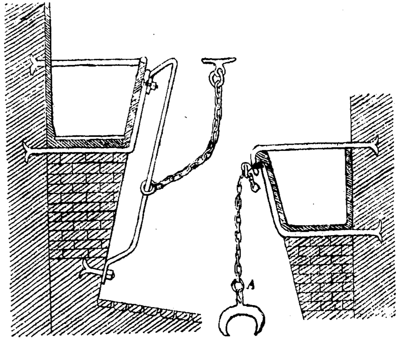
Brėž. 1 nr. Lovių įrengimas ir arklių pririšimo būdas.
