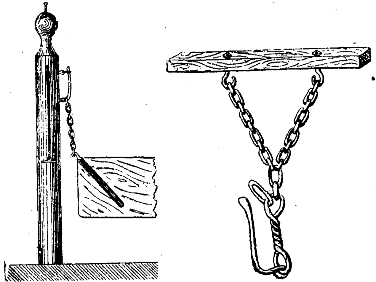
Brėž. 4 nr. Iš kairės: užpakalinis stulpas, palaikantis pertvarą; iš dešinės: dviguba grandis pertvarai pakabinti.
