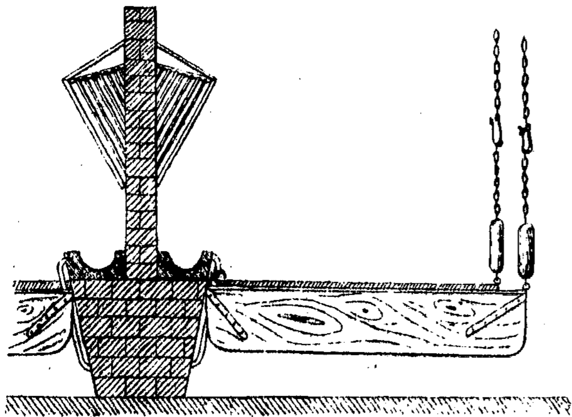
Brėž. 2 nr. Ėdžios ir pertvarų pakabinimo būdai.
