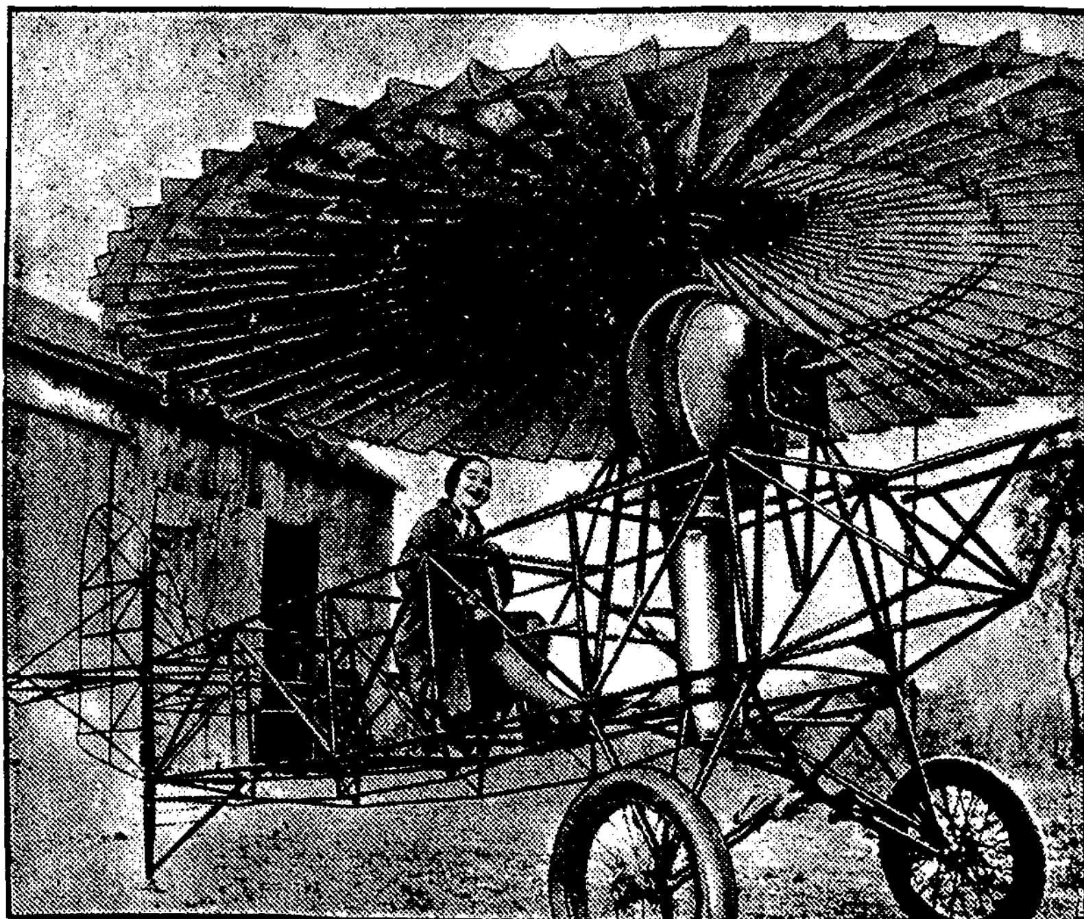
Vėl naujos konstrukcijos lėktuvas amerikiečio inž. Kindree. Šis lėktuvas gali iš visų vietų stačiai kilti į viršų.
