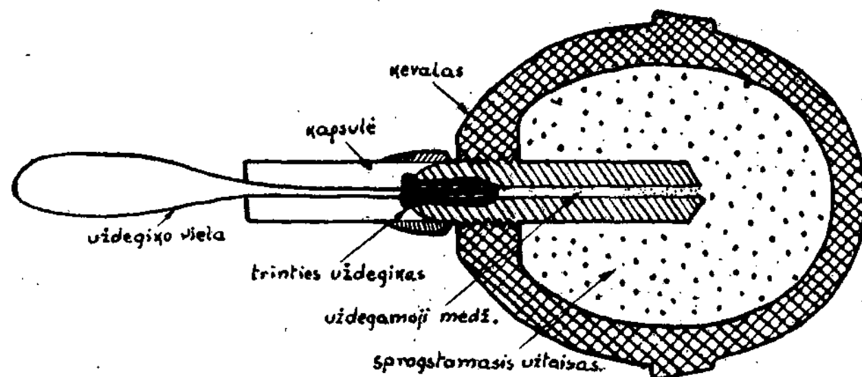
Brėž. 1 nr. Kiaušininė granata.
