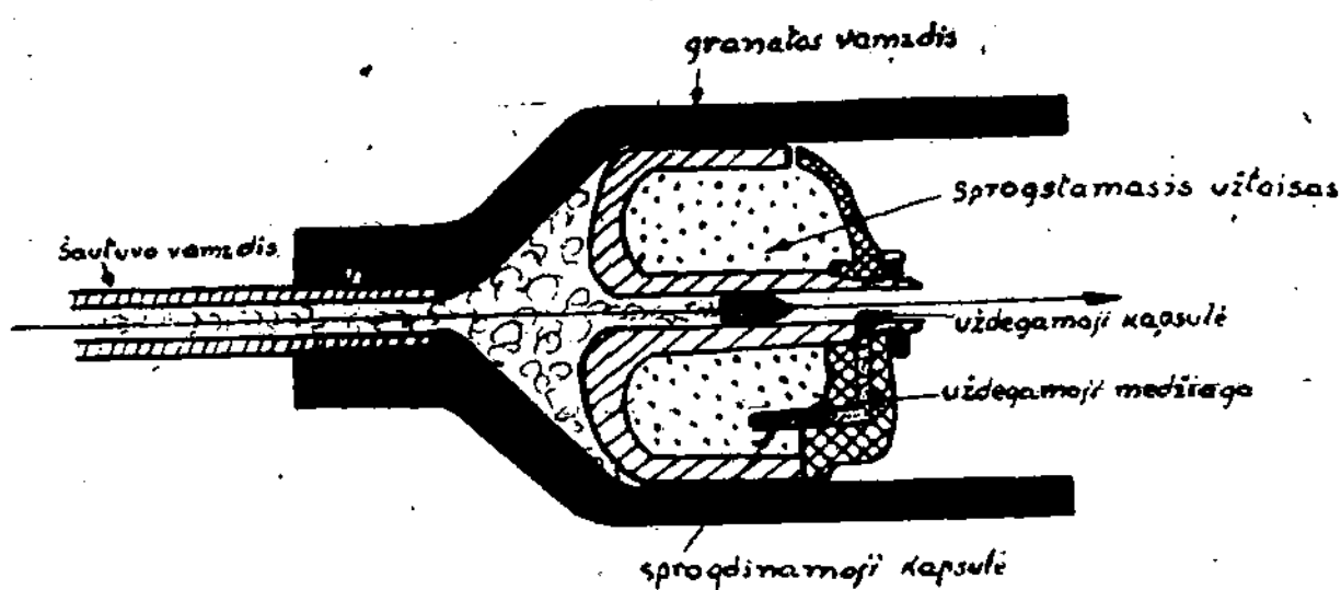
Brėž. 4 nr. Šautuvo granata.
