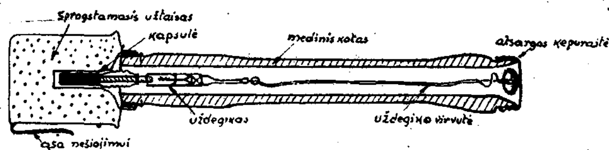
Brėž. 2 nr. Rankinė granata su koteliu.
