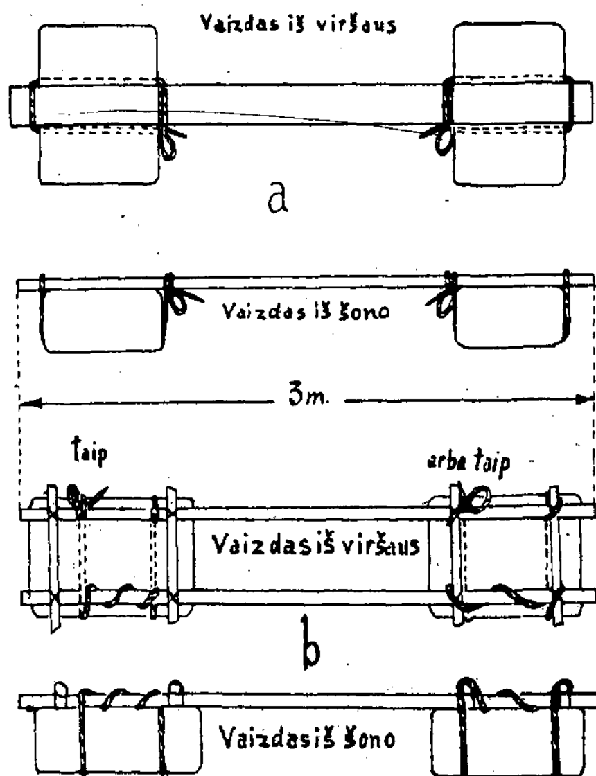
1 brėž. Plūdinio liepto atramos: a — plūdžių rišimas prie lentos; b — plūdžių rišimas prie karčių stačiakampio.
