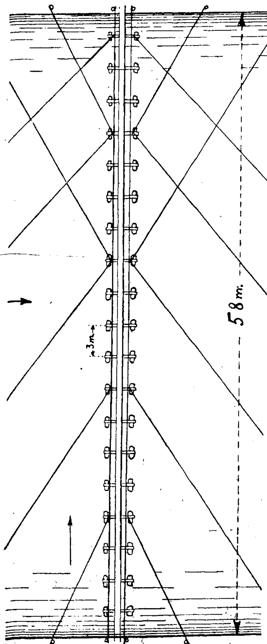
3 brėž. Plūdinio liepto perstūmimo ir pritvirtinimo schema.
