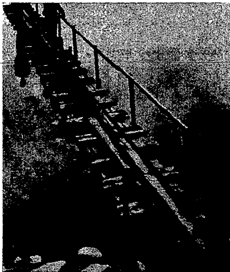
Pav. 12. Sustiprintas rąstų lieptas: dėl karčių stokos stipriną ilgesnieji basliai sukalti tik iš žemutinės pusės, prie kurių pritvirtintas vienpusis tureklis.
