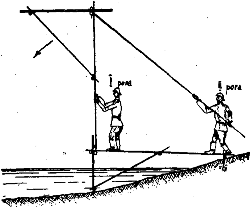
Brėž. 14. Beseler'io liepto statymas.
