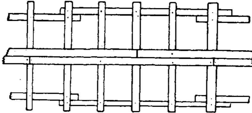
Brėž. 10. Lieptas iš vėnimis sukeltų lentų.
