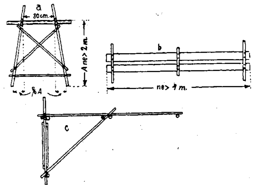
Brėž. 13. Beseler'io liepto dalių paruošimas: a — rėmas; b — skydas; c — rėmo sujungimas su skydu.
