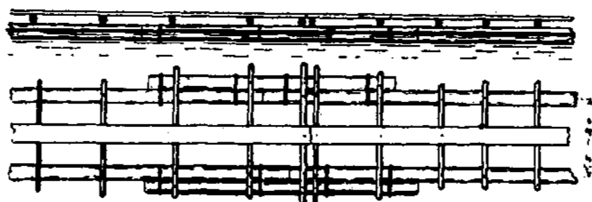
Brėž. 11. Rąstų plaukiamasis lieptas.
