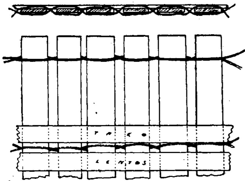
Brėž. 9. Lieptas iš plonų lentų, surištu virvėmis.
