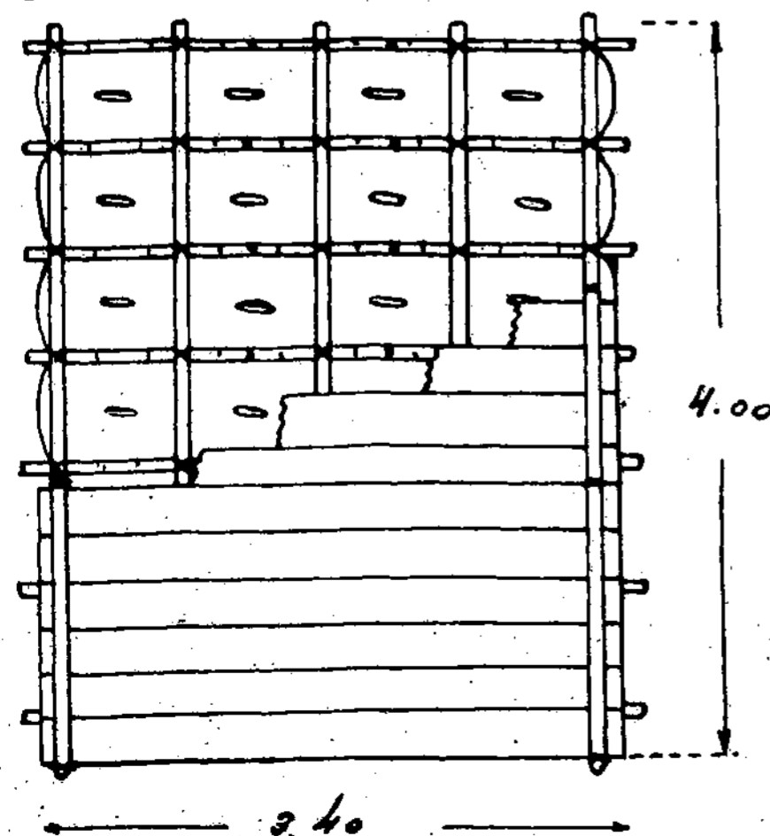
Brėž. 5. Plūdžių keltas žmonėms kelti iš karčių ir lentų.
