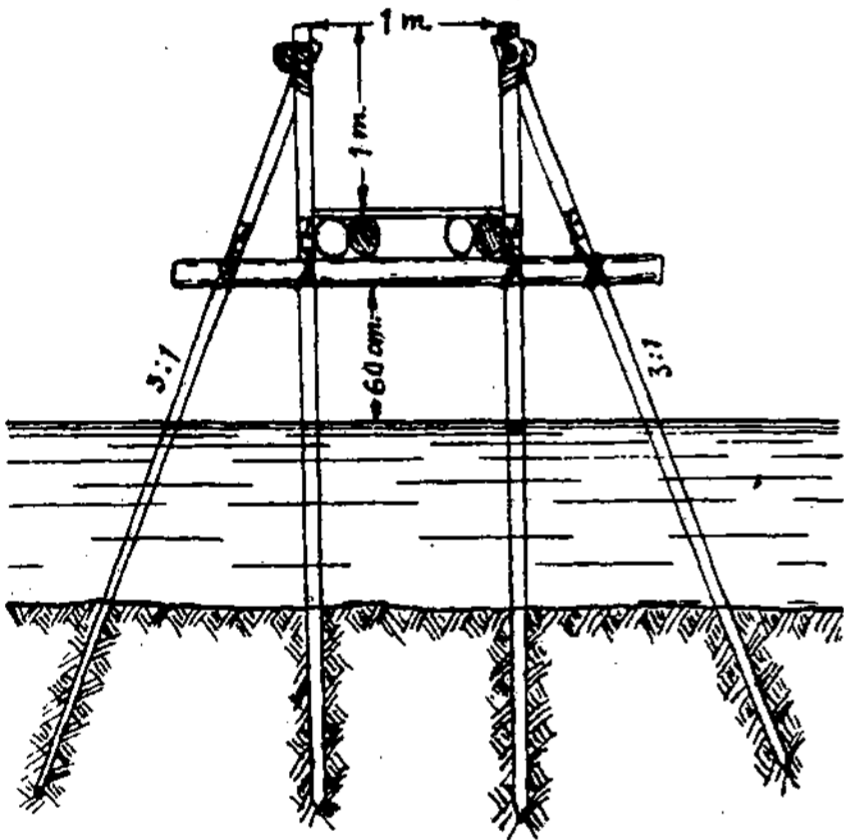
15 br. Polinio liepto atrama.
