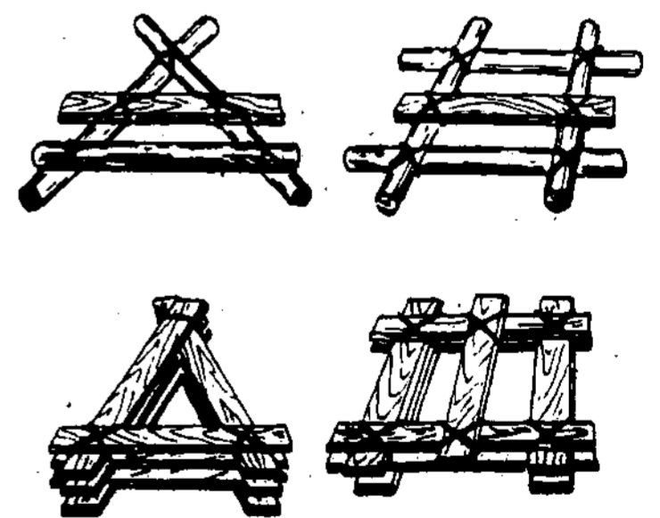
Brėž. 18. Rastų ir lentų kelteliai.
