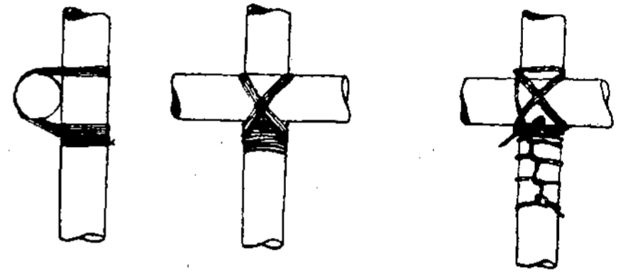
Brėž. 16. Skersinio pririšimas prie polio ir spyrio virve.
