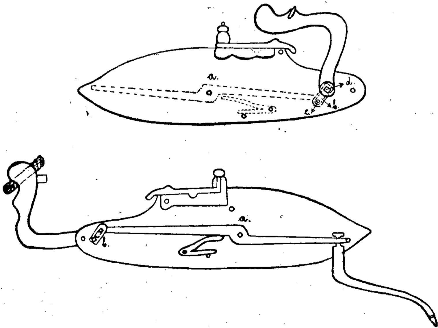
Brėž. 2. Knatinė spyna.
