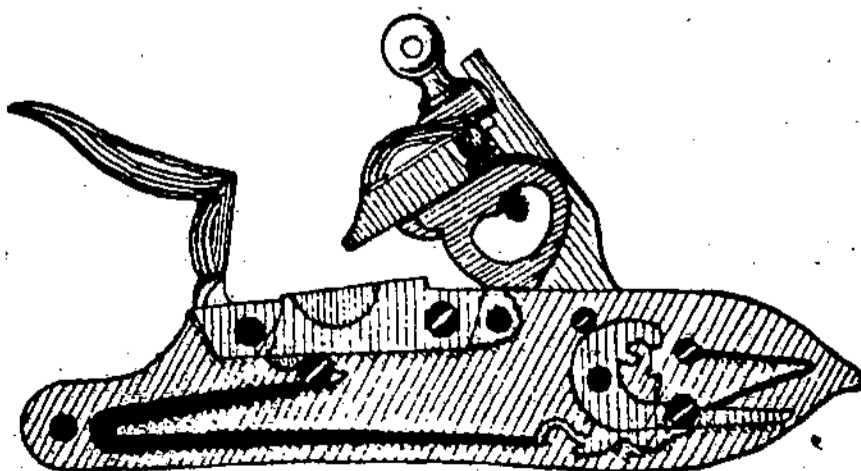
Brėž. 6. Skiltuvinė spyna.
