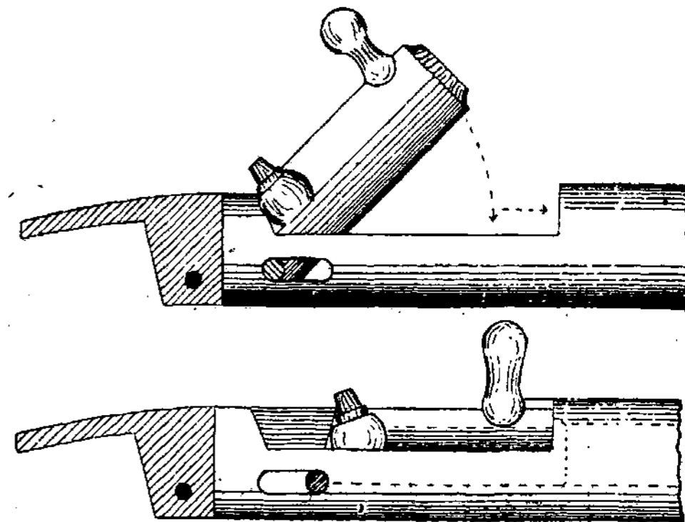
Brėž. 12. Uždaras, užtaisantis per drūtgalį.
