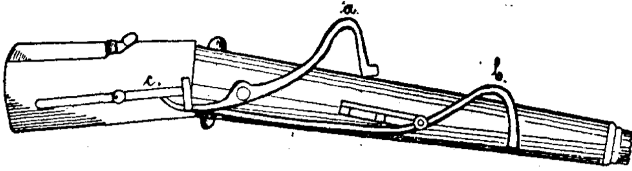
Brėž. 3. Patobulinta knatinė spyna.
