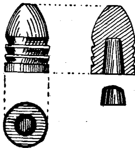
Brėž. 11. Pailgoji kulka.
