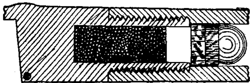
Brėž. 9. Apvali kulka.
