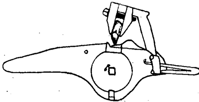
Brėž. 5. Ratinė spyna.
