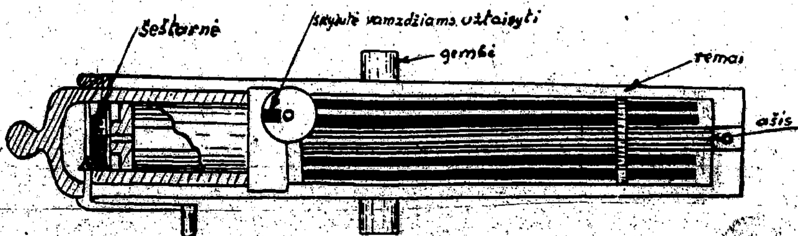
Gotlingo kartečinė. Viršuj brėž. 4 (kartečinės vaizdas iš šono) ir apačioj brėž. 5 (jos vaizdas iš viršaus).
