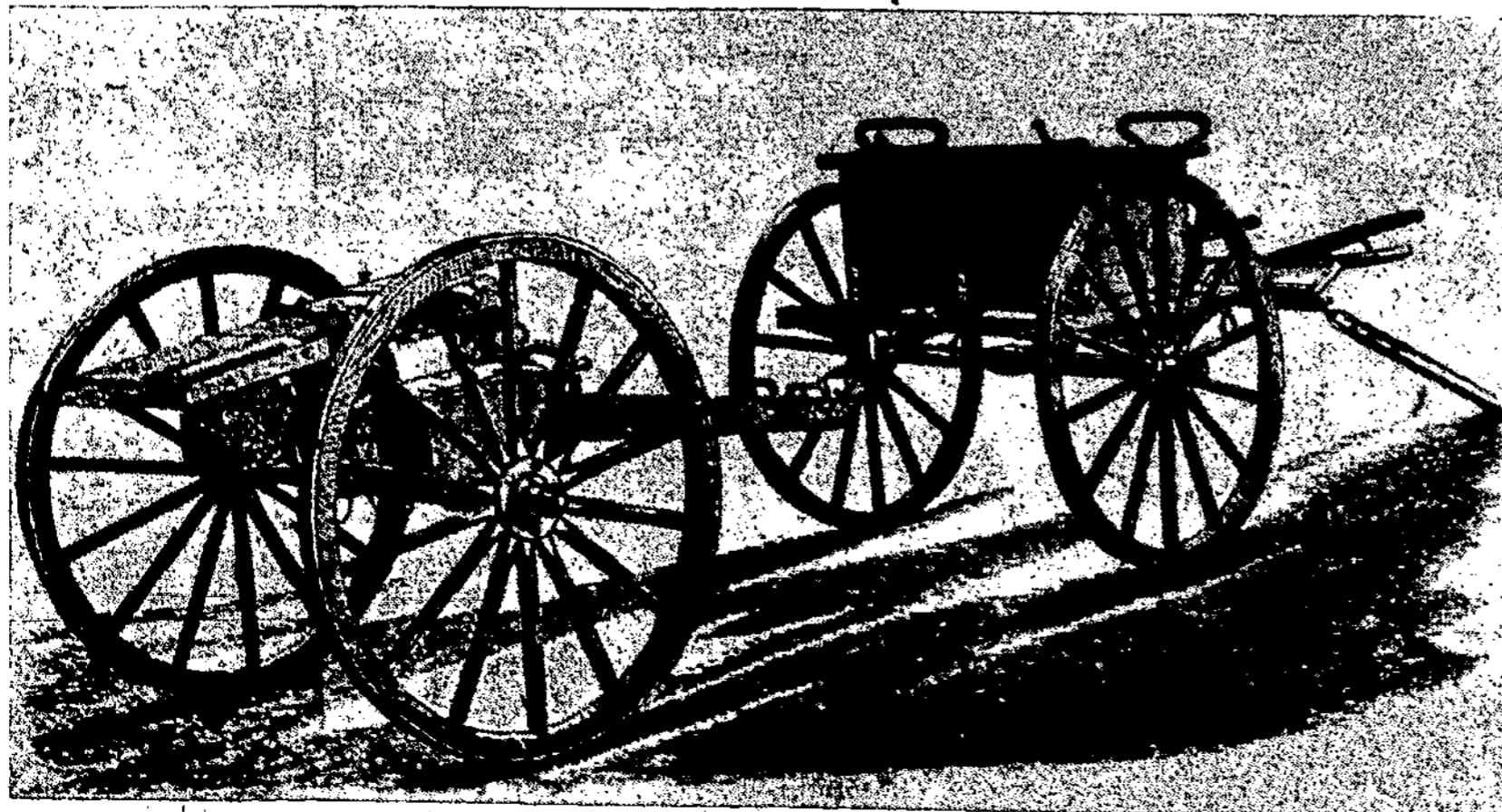
Pav. 8. Nordenfeldo kartečinė (10 vamzdžių) su pirmagaliu.
