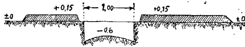
Brėž. 4. Melagingas šaulių apkasas.
