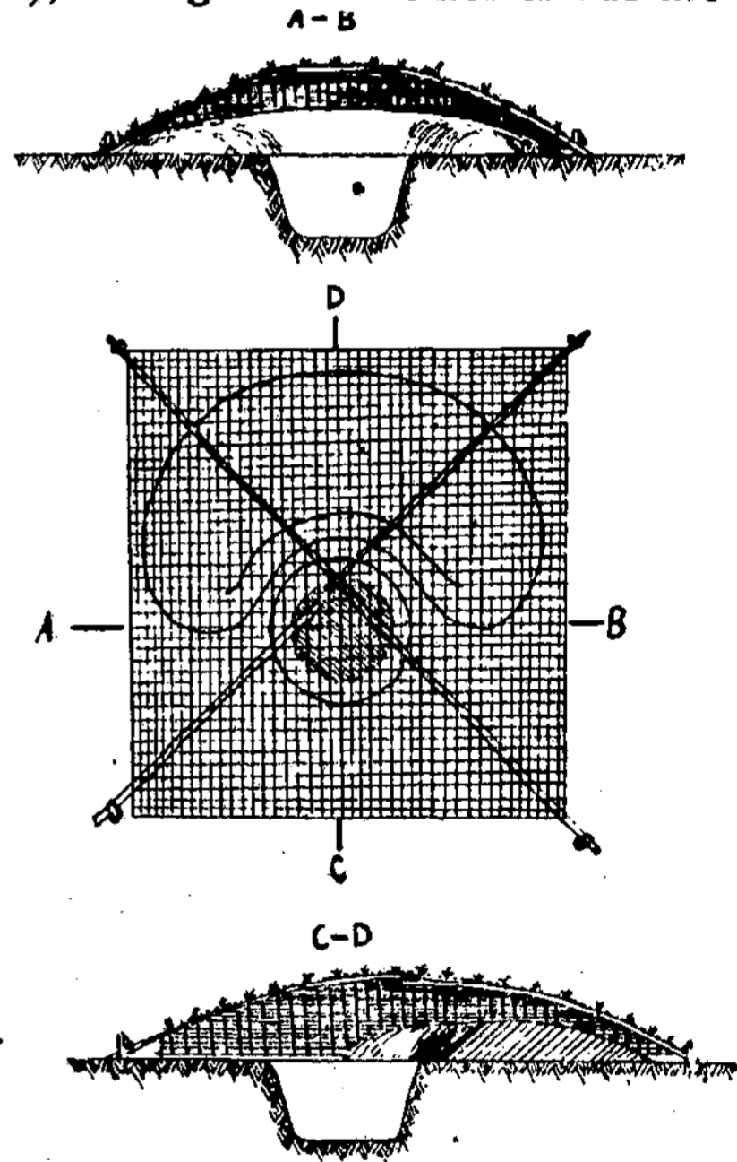
Brėž. 8. Tinklais maskuoti apkasal.
