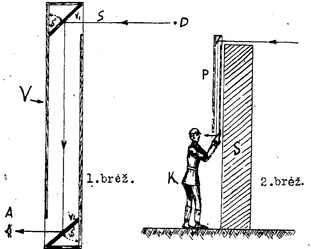
1. brėž. Veidrodinis periskopas: V — vamzdis; V^1 , V^2 — veidrodėliai; D — daiktas; S — spindulys; A — sekėjo akis.
