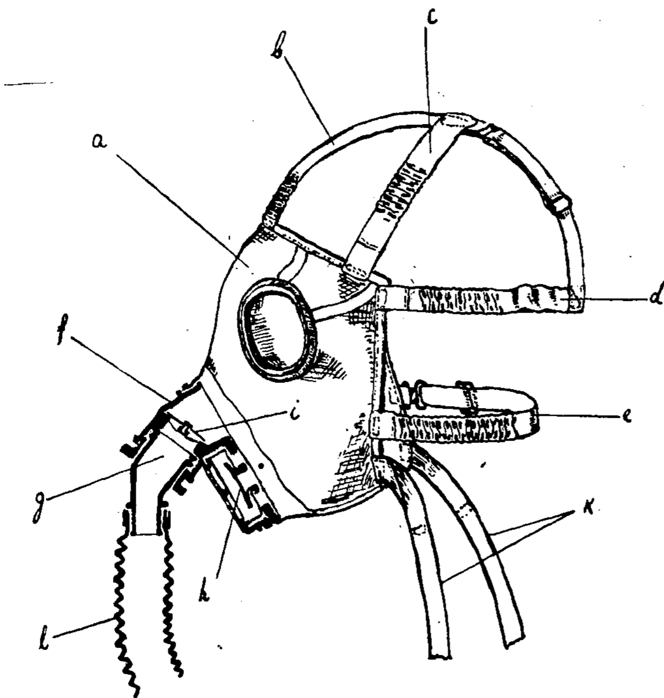
Br. 1. Kaukė ir vožtuvų dėžutės piūvis: a) kaukės gumuotas audeklas, b) kaktos raikštis, c) smilkinių raikštis, d) pakaušo raikštis, e) sprando raikštis, f) vožtuvų dėžutė, g) kvėpavimo anga, h) iškvėpiamasis vožtuvas, i) įkvėpiamasis vožtuvas, k) kaukės kaspinas, l) kvėpavimo žarna.
