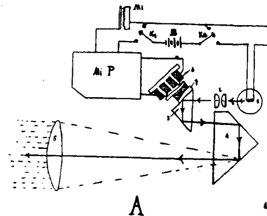
Principinė optinio telefono schema
