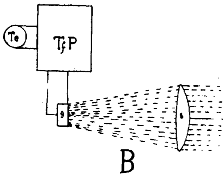
Principinė optinio telefono schema
