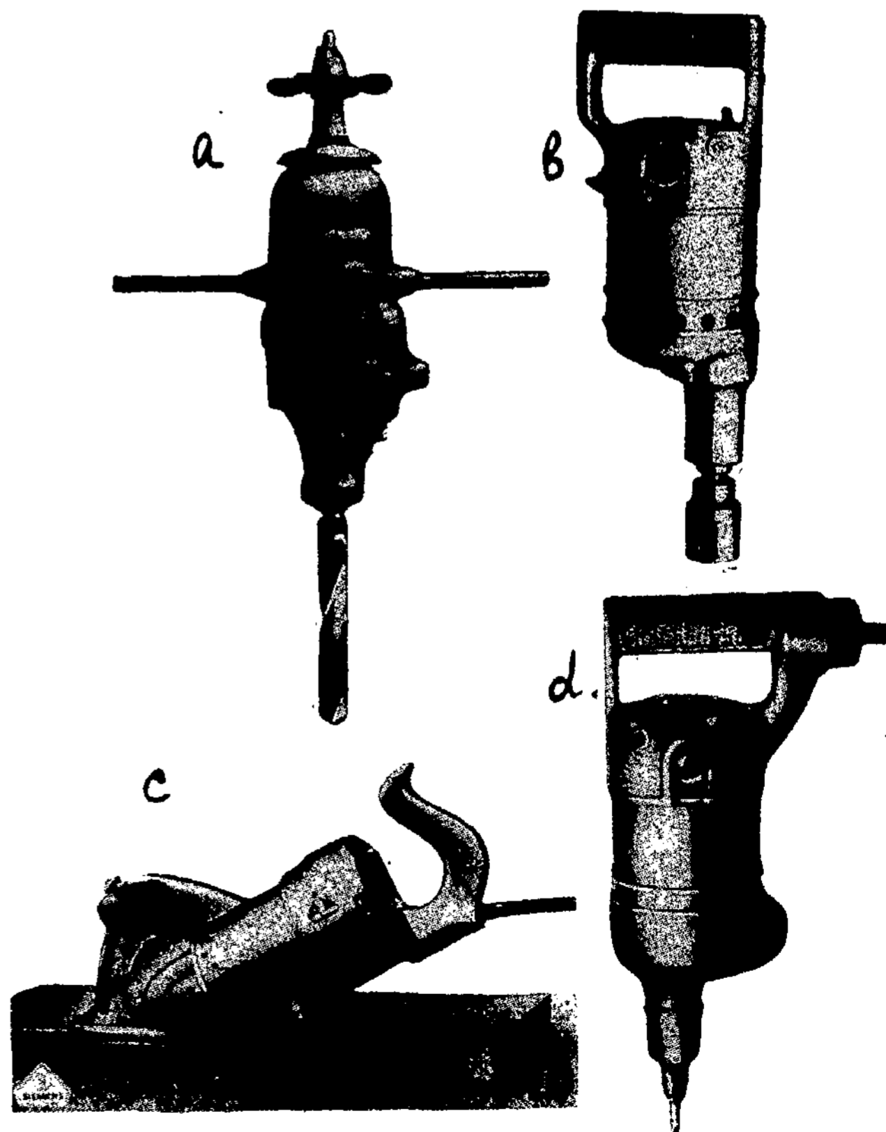
2. brėž. Elektriški įrankiai: a — grąžtas skylėms 23 — 100 mm dm. gręžti; b — grąžtas skylėms 4 — 30 mm; c — apskritas piūklelis; d — atsuktuvai.
