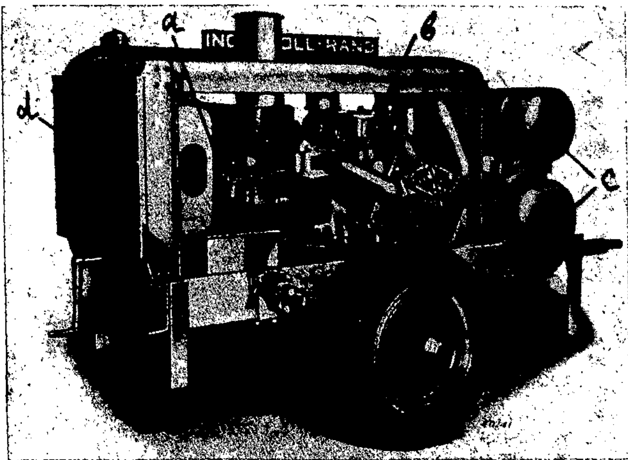
Kilnojamas kompresorius: a — vidaus degimo variklis; b — kompresorius; c — oro rezervuarai; d — radiatorius.
