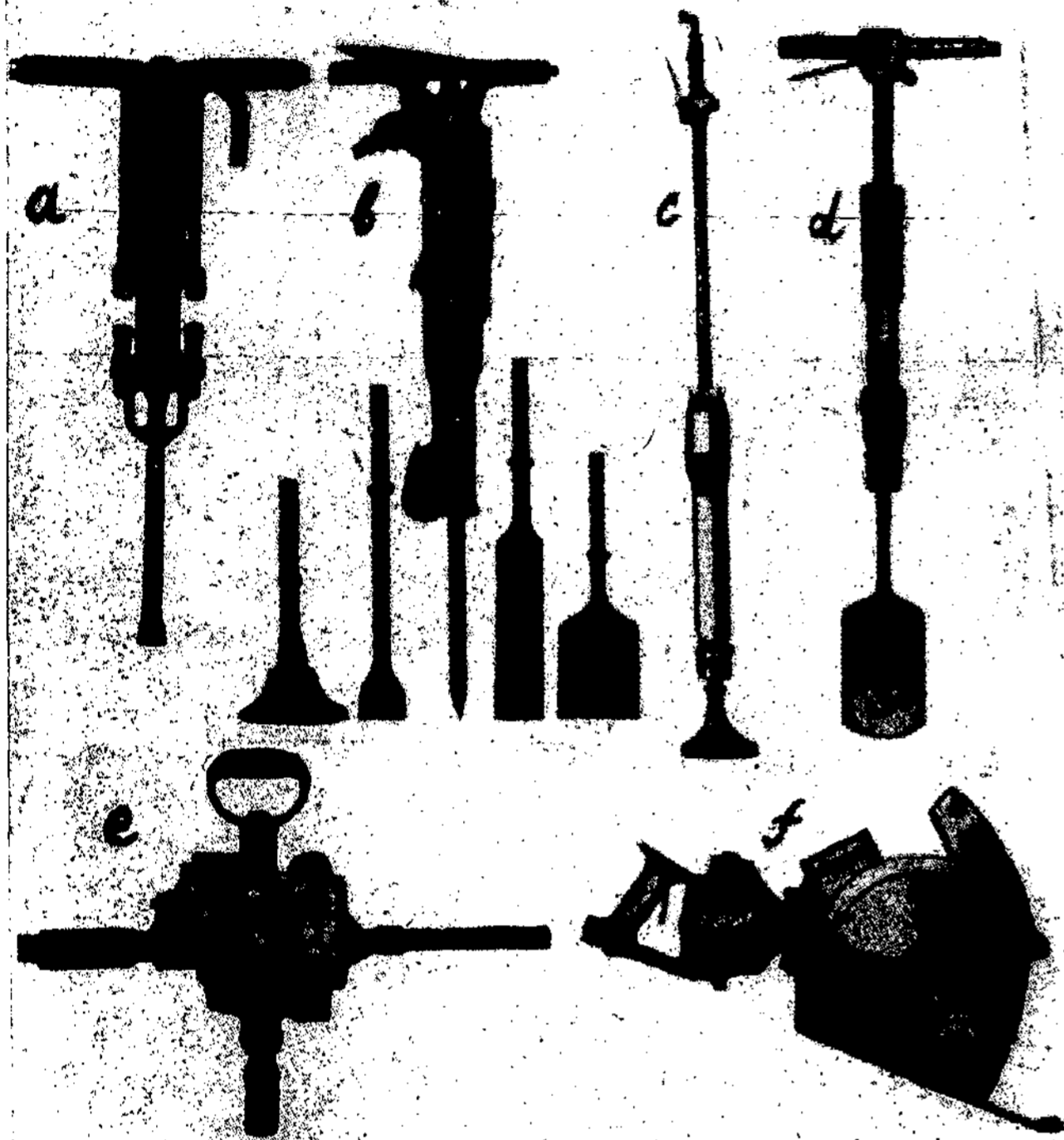
1. brėž. Pneumatiniai įrankiai: a — akmens kaltas — grąžtas; b — dalba su kitokių įrankių galais, į ją įstatomais; c — pluktuvas; d — kastuvas; e — grąžtas medžiui ir vidutiniam gruntui gręžti; f — apskritas piūklelis.
