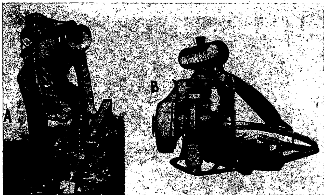
3. brėž. A — medžio gręžimas individualaus motoro pagalba; B — individualus motoras įvairiems pionierių įrankiams varyti.
