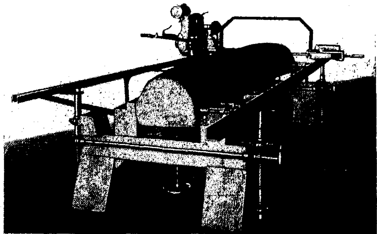
Sudedamosios staklės motoriniu piūklui išilgam medžio piovimui
