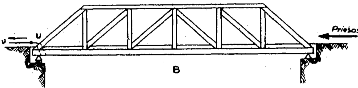
Br. 5. Tiltų sprogdinimas su vienu užtaisų vienoje tilto pusėje: U — užtaisai; V — viela arba virvė, priišta prie dviejų granatų degtuvų virvelių.
