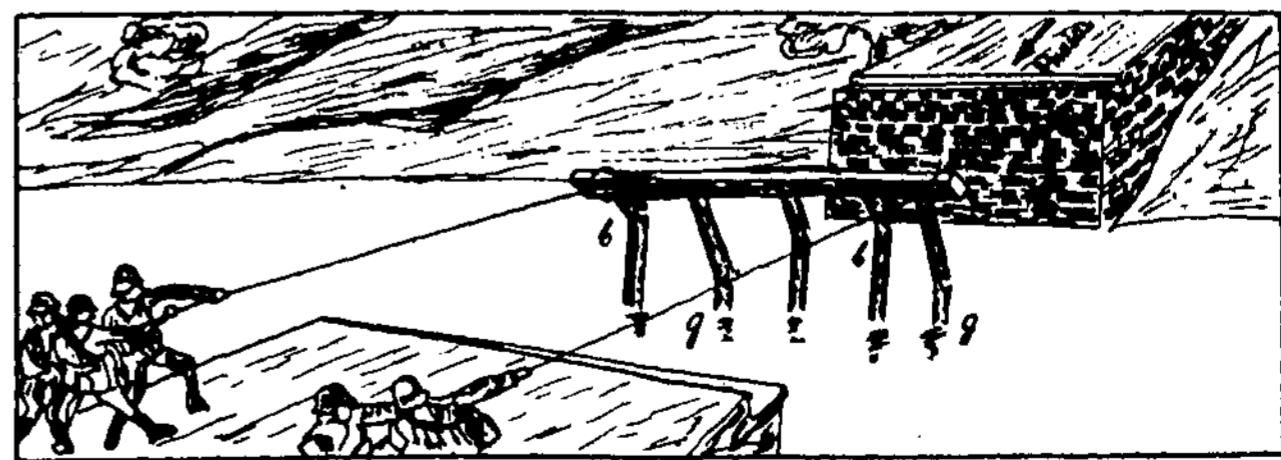
Br. 2. Tilto pakirstos atramos nulaužimas: b — peraugštai įkirsti poliai — blogai; g — gerai.
