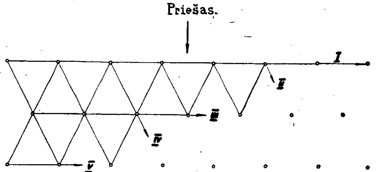
10 brėž. Darbo schema apraizgant spygliuota viela baslius: I, II, III, IV ir V — žmonių trejukų (dvejukių) vietos su vielos kamuoliais. Pirmoje eilėje viela kalama iš priešos pusės; tarp eilių prie pirmos eilės iš vidaus, prie antros iš priešos; antroje ir trečioje eilėje — iš savo pusės.
