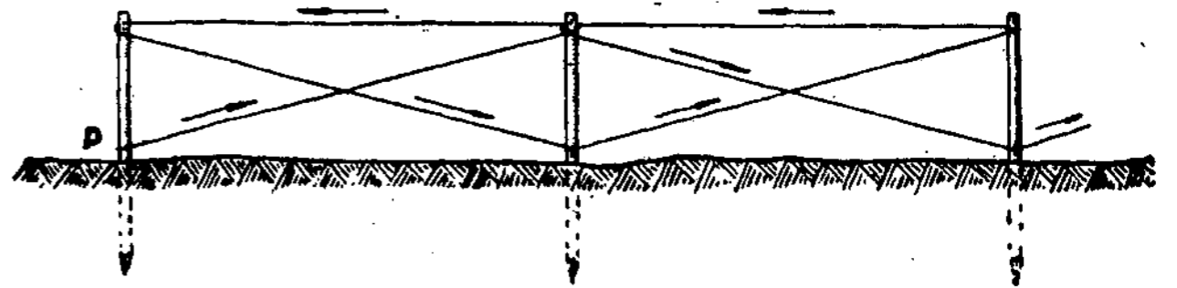
9 brėž. Eilių ir tarpų apraizgymo tvarka: strėlė rodo vielos tiesimo kryptį, p — pradžia.
