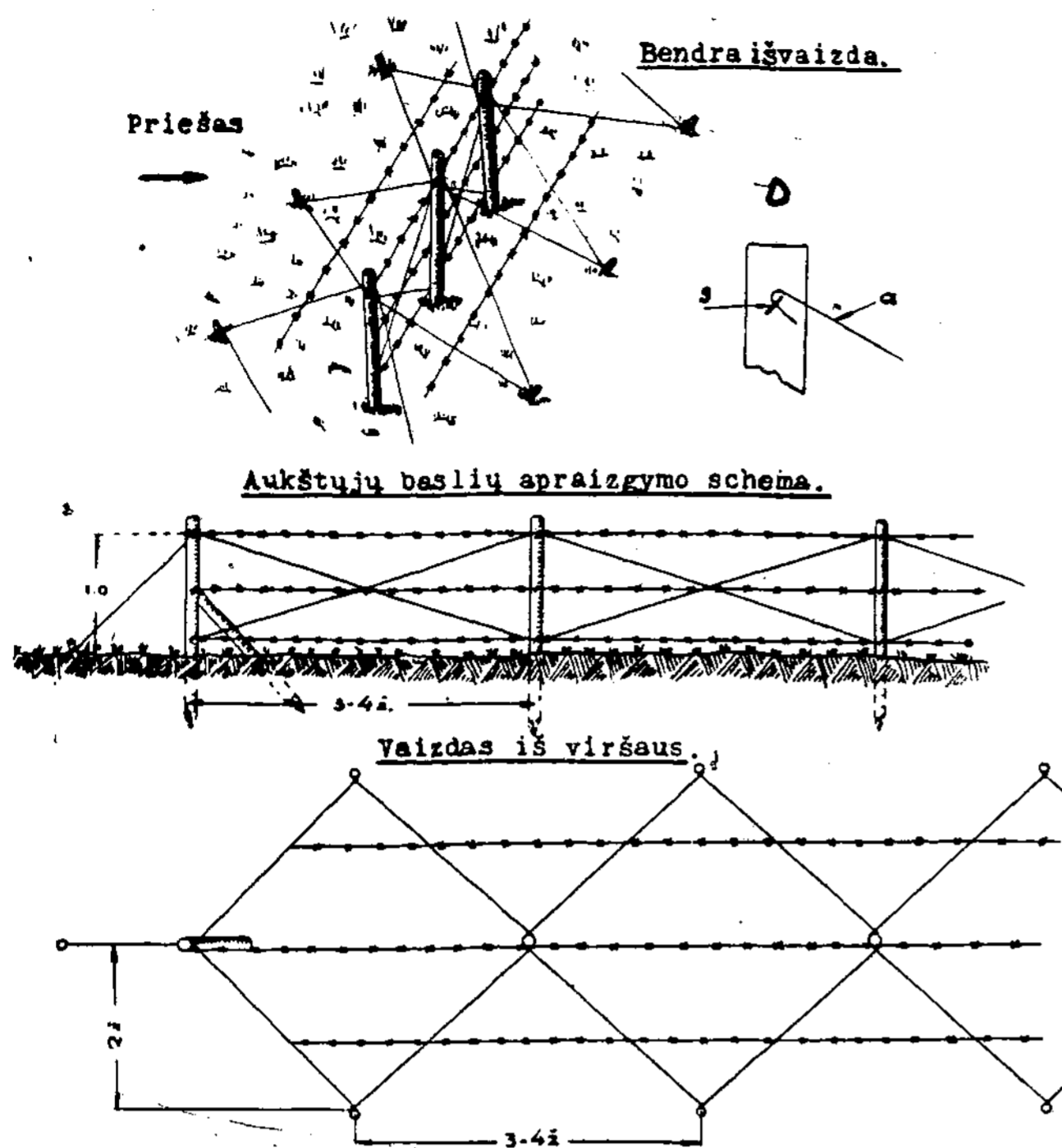
3 brėž. Vielinė tvora. D — atasijos pritvirtinimas prie baslio; a — atasija; s — sankabėlė.
