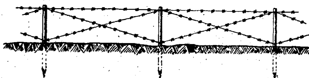
7 brėž. Normaliojo tinklo antrųjų eilių ir tarpų raizgymas
