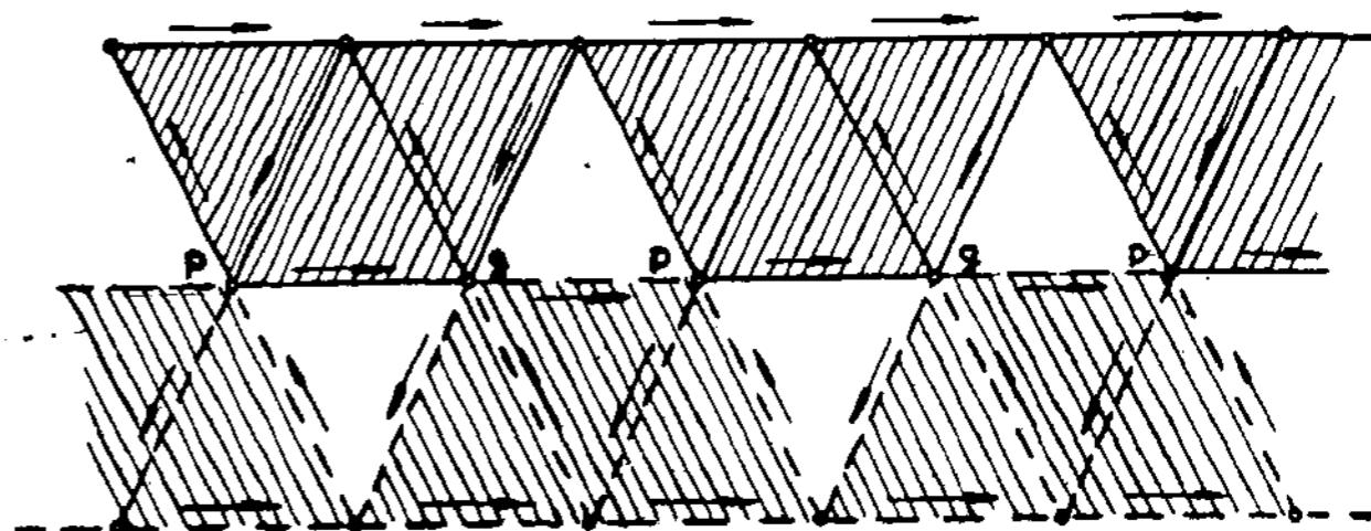
5 brėž. Dviejų grupių darbo schema apraizgant žemojo tinklo baslius: ištisinė linija — I grupės viela, p — pradžia, g — pabaiga; taškuota linija — antros grupės viela, g — pradžia, p — pabaiga. Grupė padarius trapeciją iš trijų trikampių kerpa vielą ir pereina prie kitos trapecijos.
