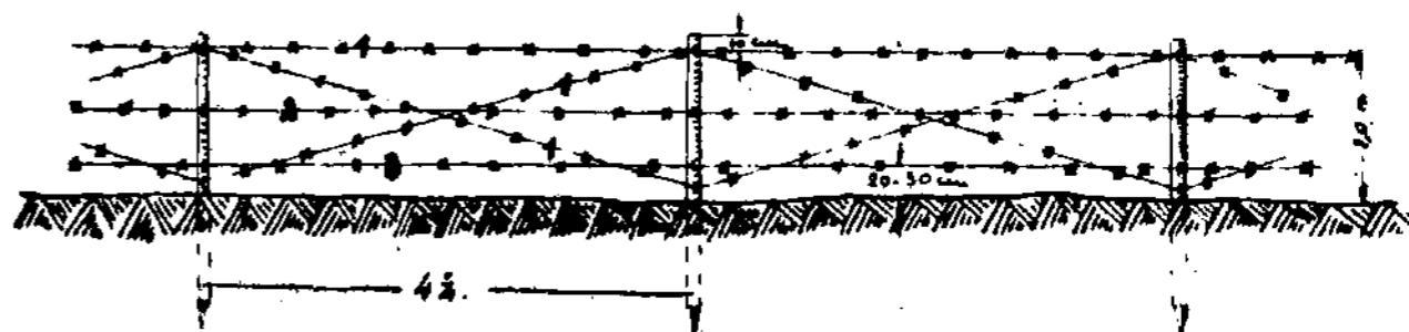
6 brėž. Priekinė normaliojo tinklo eilė.
