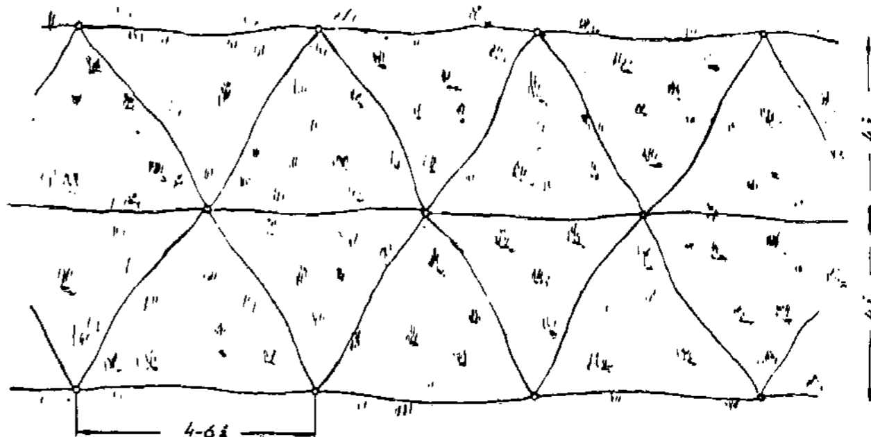
4 brėž. Žemasis vielinis tinklas; s — spyralė.
