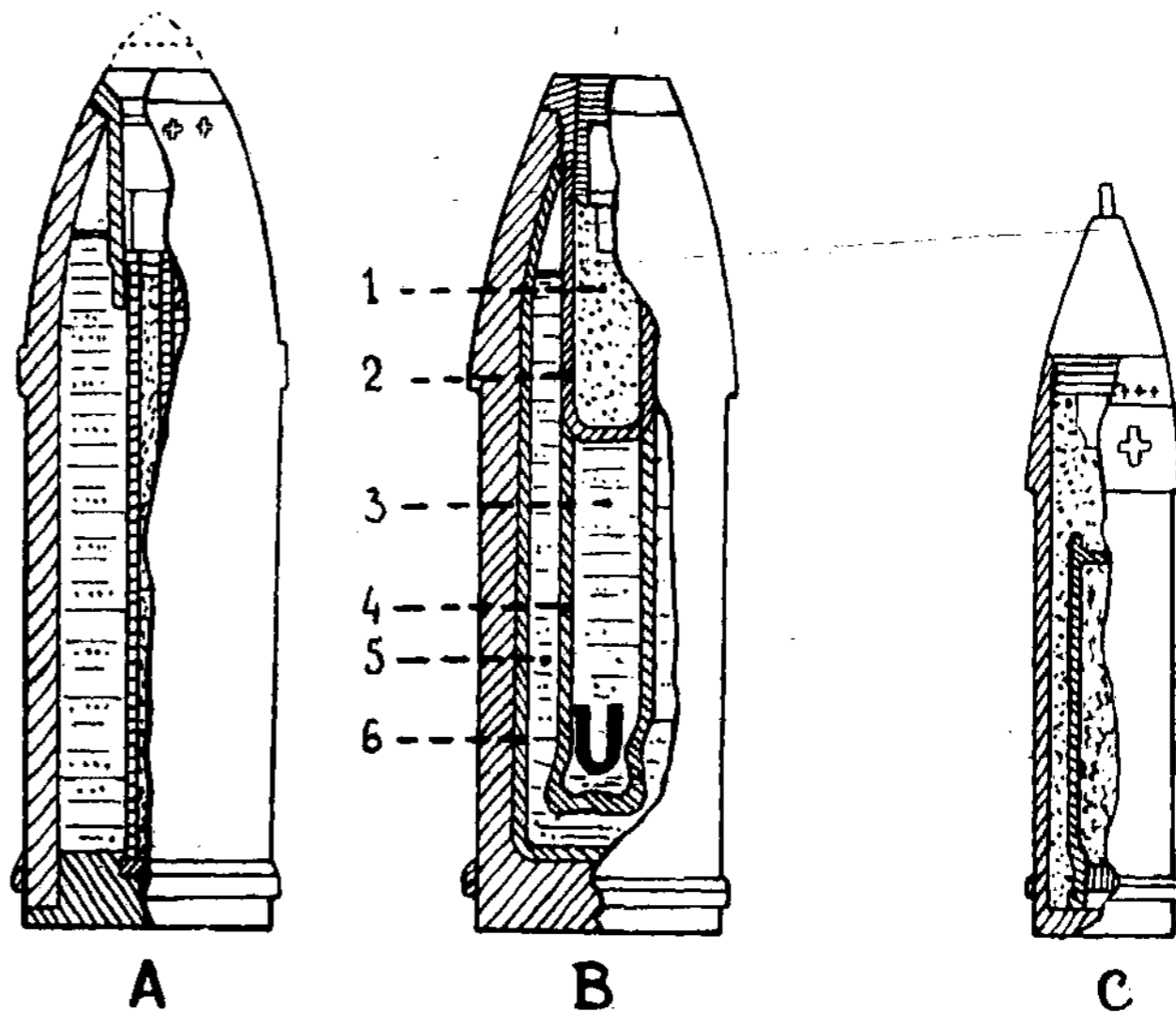
Dujiniai sviediniai. A ir B užtaisyti su dujų skysčiais, C — su sausais kristalais.
