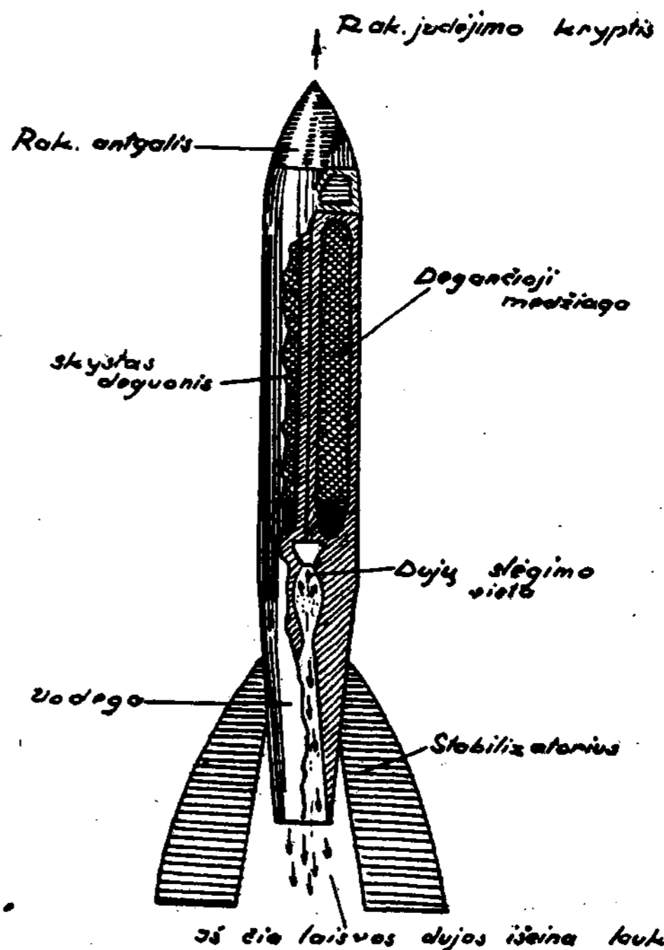
4 brėž. Viena šių dienų stambiųjų raketų
