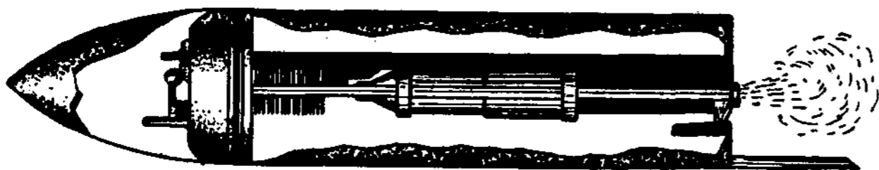
3 brėž. Goddardo raketa tarpplanetiniam skridimui
