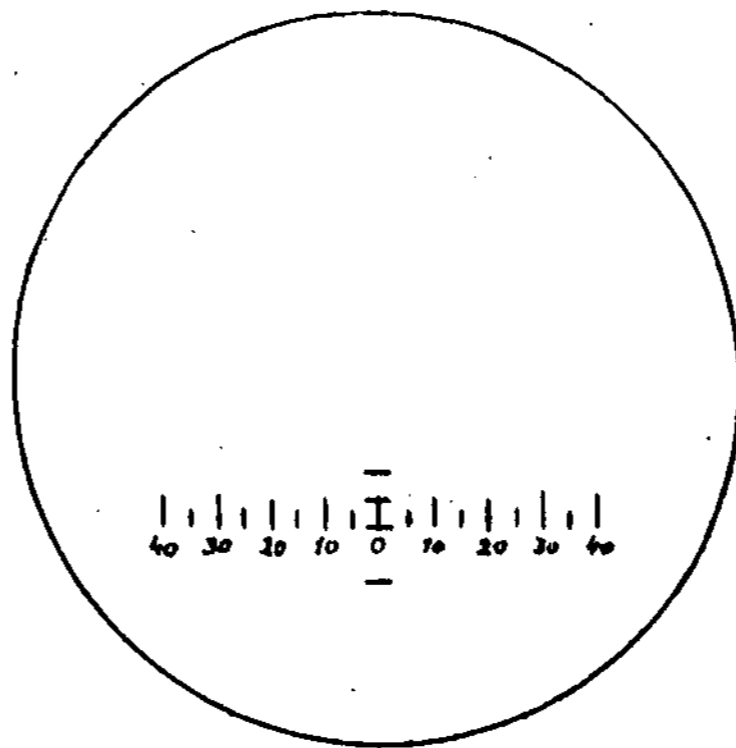
2 brėžinys. Dviejų tipų žiūrono tinklelis
