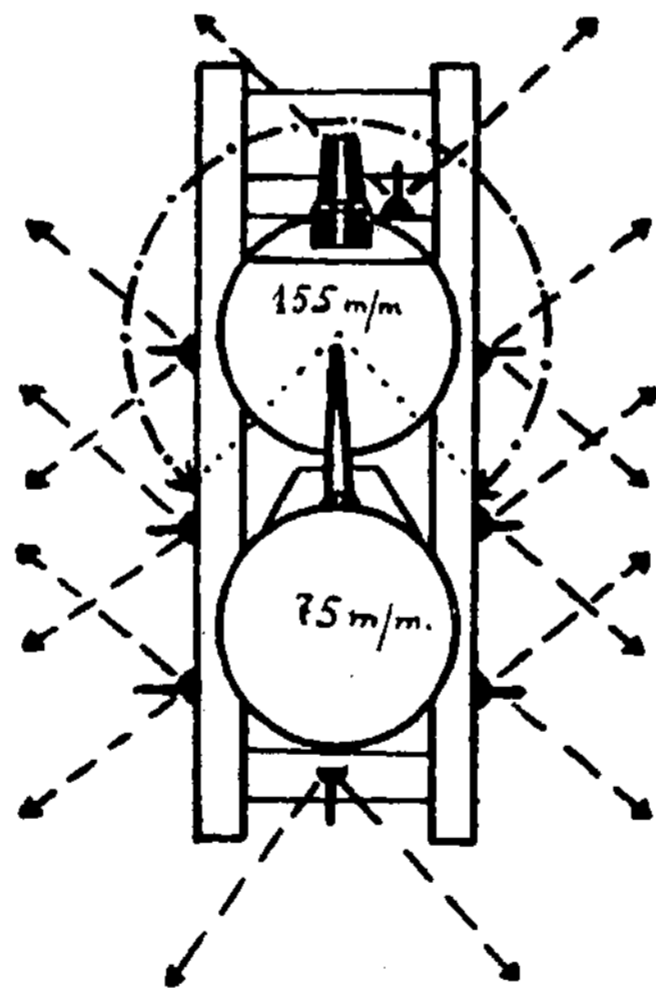
3 schema. Prancūzų sunkusis tankas, ginkluotas 8 kulkosvaidžiais, vienu 155 mm pabūklu, šaudančiu 280^\circ kampu ir vienu 75 mm pabūklu, šaudančiu 360^\circ kampu
