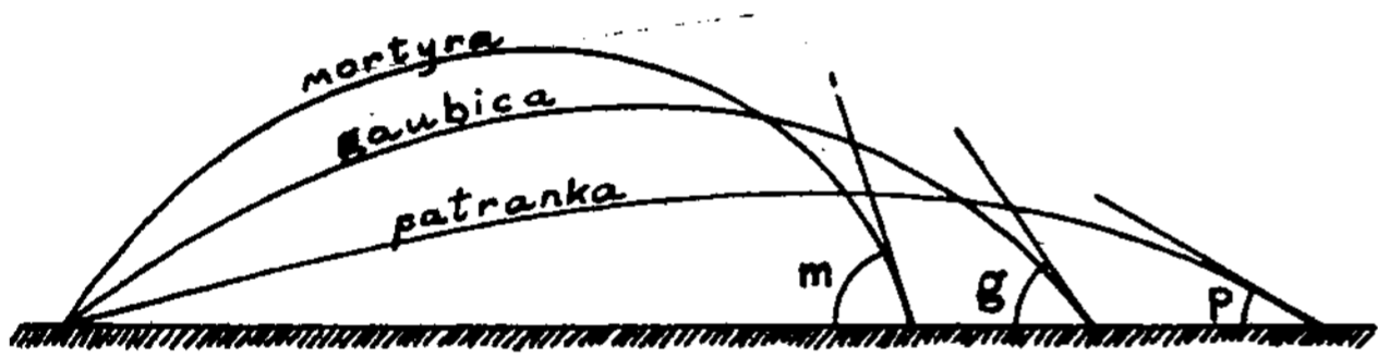
9 br. Kritimo kampai: m — mortyros, g — gaubicos ir p — patrankos
