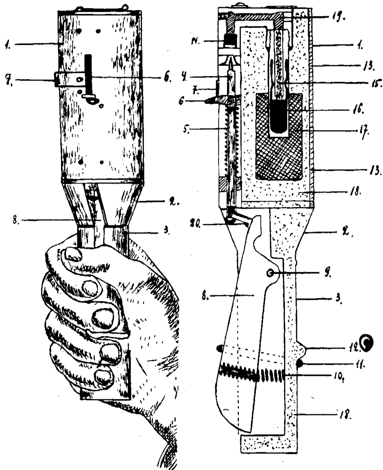
1 brėž. Rusų 1914 m. pavyzdžio rankinė granata
