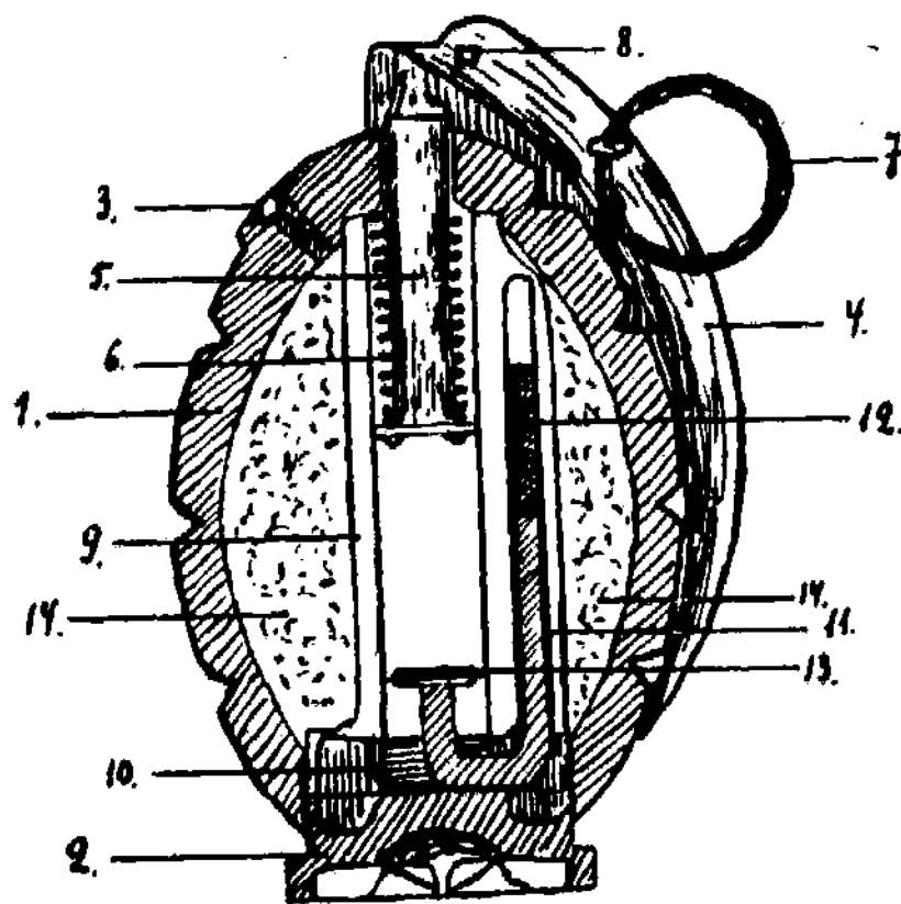
Anglų Mills'o sistemos rankinės granatos piūvis
