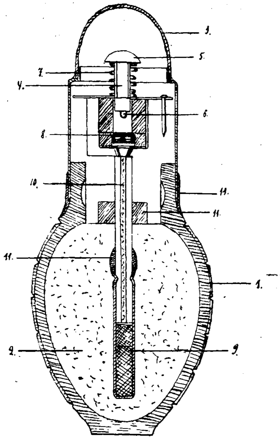
Prancūzų rankinės granatos „C. F.“ piūvis
