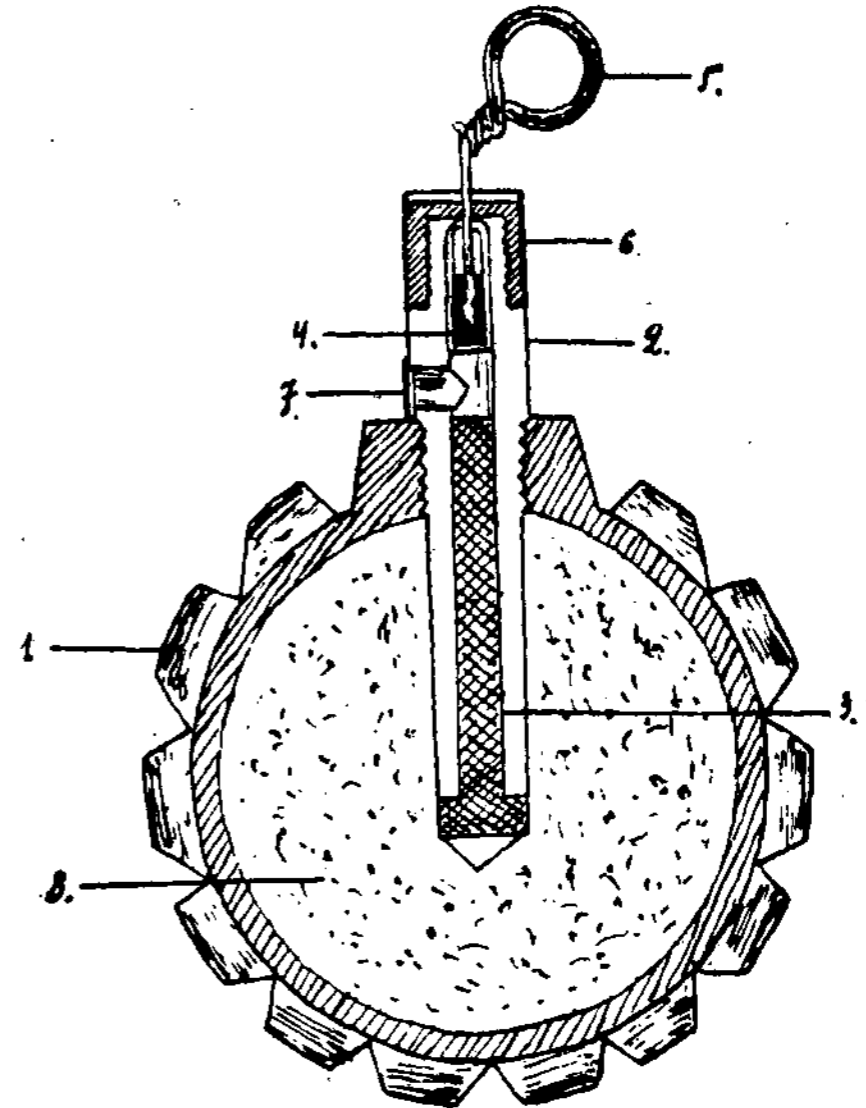
Rutulinės granatos piūvis
