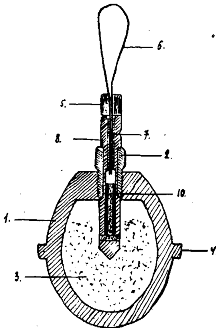
Kiaušininės granatos piūvis
