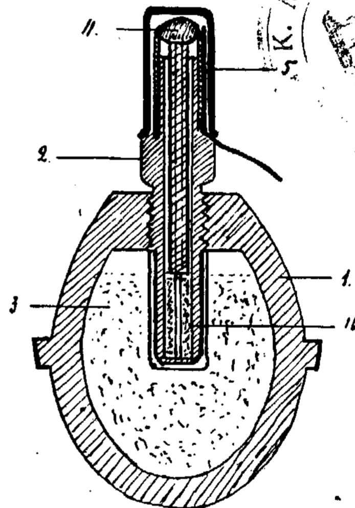
Kiaušininės granatos piūvis kitos rūšies degtuvu
