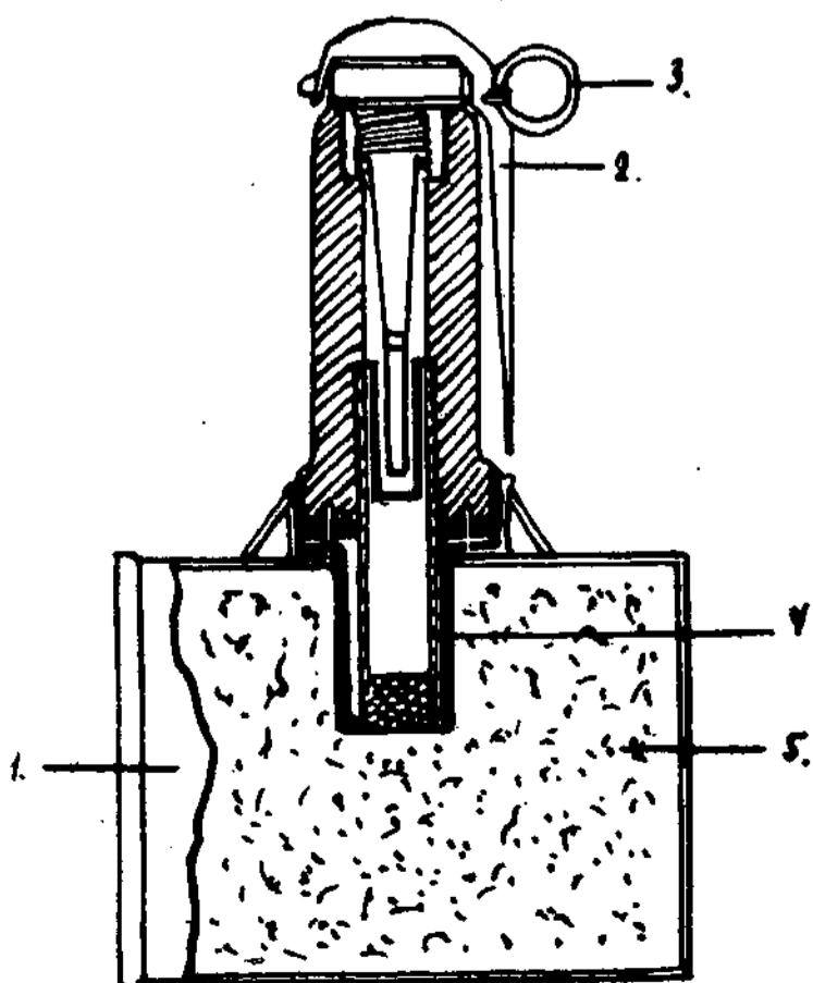
Prancūzų rankinė prieštankinė granata
