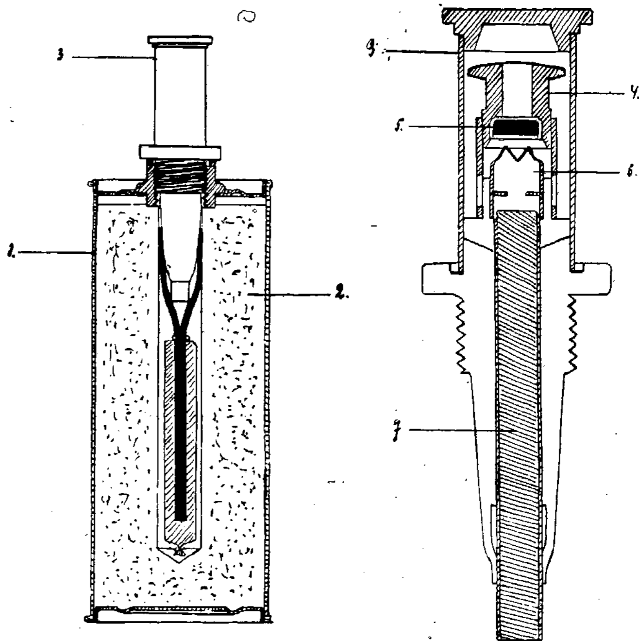
Prancūzų 1916 m. pavyzdžio uždegamosios rankinės granatos piūvis
