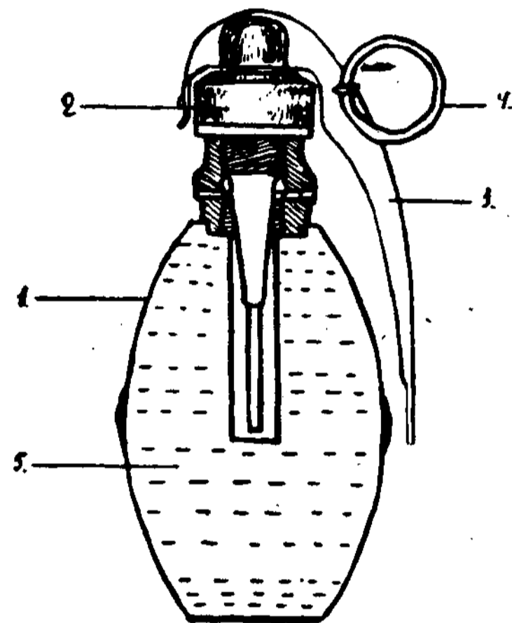
Prancūzų 1916 m. pavyzdžio rankinės dujinės granatos piūvis
