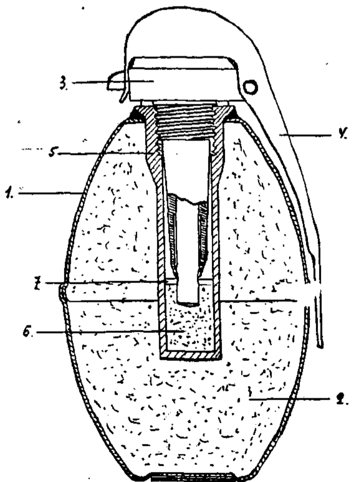
Prancūzų 1916 m. pavyzdžio uždegamosios rankinės granatos piūvis
