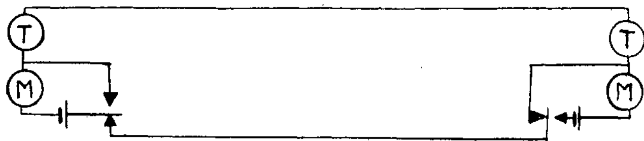
10 brėž. Dvipusė telefono ir mikrofono schema
