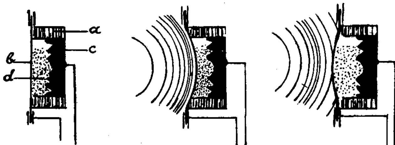
9 brėž. Mikrofonas: a — dėžutė (nelaidi), b — membrana, c — anglinė kaladėlė, d — angliniai grūdėliai. 9a ir 9b brėž. Mikrofono virpėjimai kalbant.
