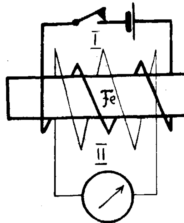
11 brėž. Indukcinė ritė
