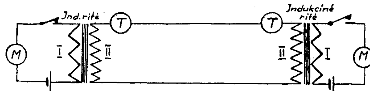
12 brėž. Dvipusė telefono ir mikrofono patobulinta schema (su indukcinė rite)
