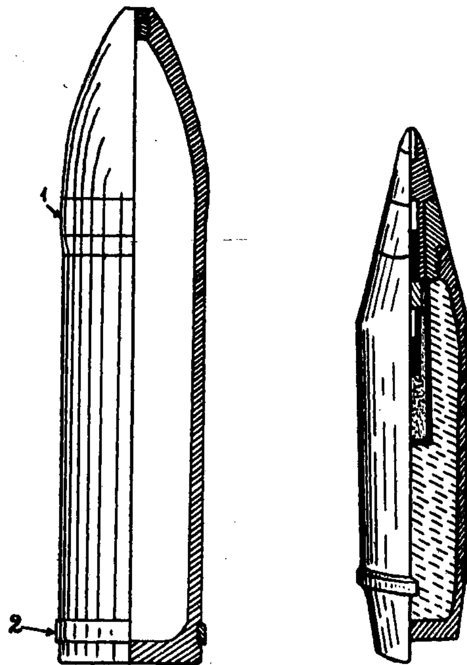
1 pieš. 1 — centruojamoji storuma 2 — vedamasis žiedas
