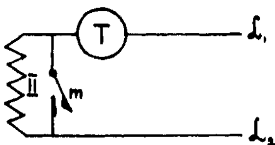
13 brėž. Indukcinės ritės II apvijos šuntavimas (klausant nuspaudžiamas mygtukas m)
