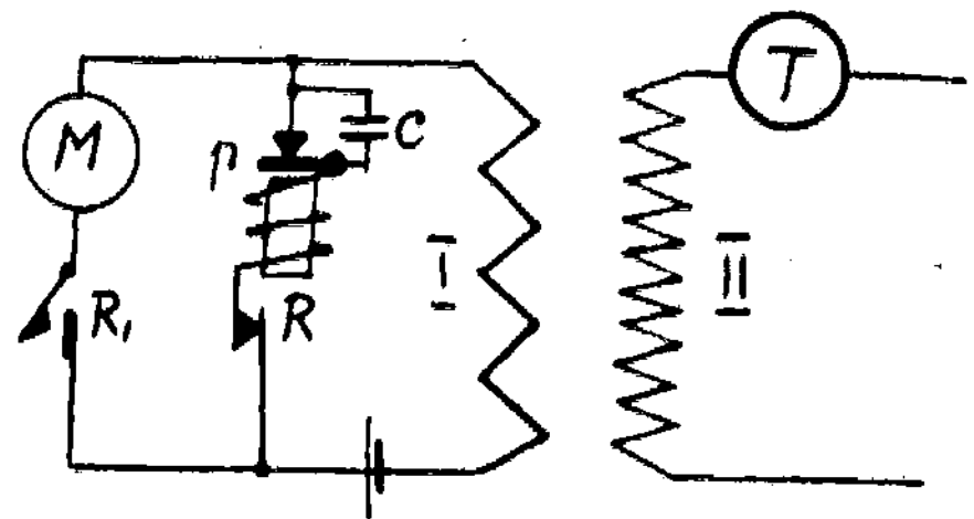
15 brėž. Zirzeklio principinė schema
