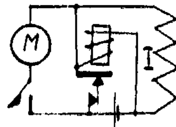
17 brėž. Zirzeklio ritė įjungta lygiagrečiai indukcinė ritei
