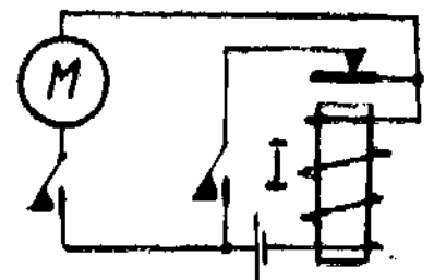
18 brėž. Zirzekliui panaudota indukcinės ritės pirminė špūlė
