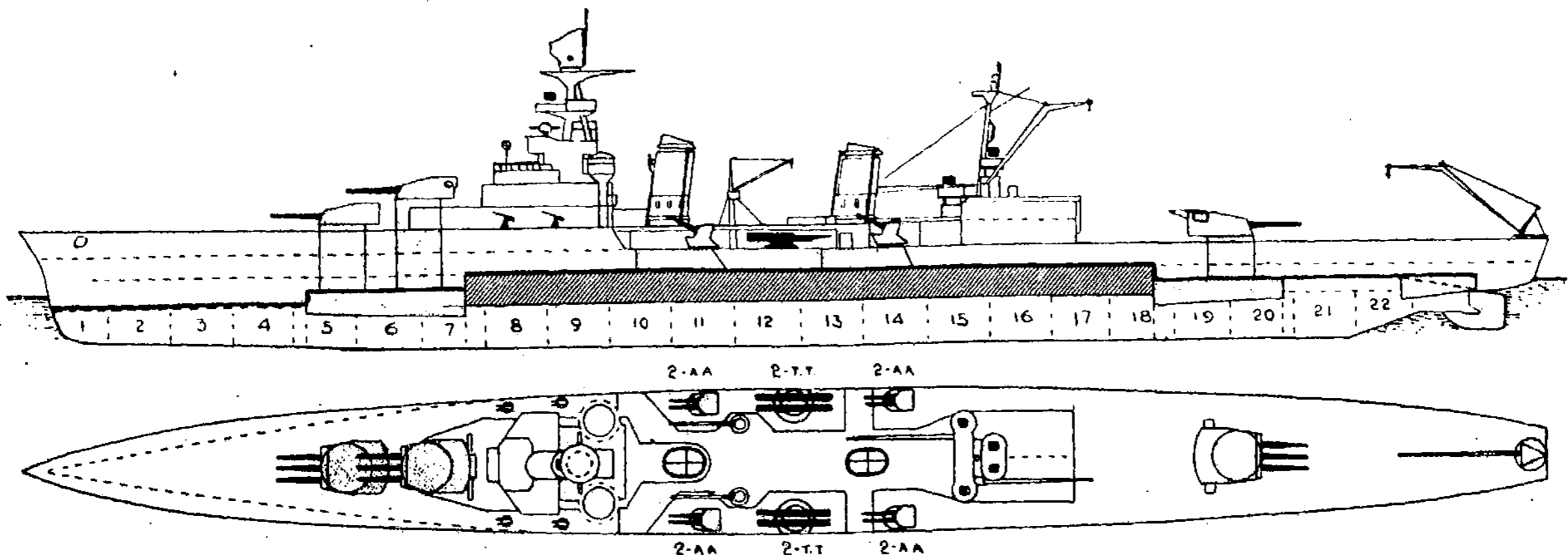
Prancūzų lengvojo kreiserio „La Galissonnière“ vaizdas iš šono ir iš viršaus. Kreiseris yra 1933 m. statybos, 7600 tonų, 184 m ilgio ir 17 m pločio. 88.000 a. j. varomas plaukia iki 35 jūrmylių (63 km) per val. Jo apginklavimą sudaro: pagrindinė artilerija — 9 pabūklai 152 mm, 50 kalibrų ilgio, antros eilės artil. — 8 priešlėktuviniai 90 mm pabūklai ir treč. eil. artil. — 8 priešlėktuv. 37 mm automatiniai pabūklai, 4 torpedoms leisti 533 mm aparatai ir 4 lėktuvai. Šarvai nuo 95 iki 140 mm storio. Jie schemoje pažymėti tamsiau. Laivo įgulą sudaro 608 žmonės
