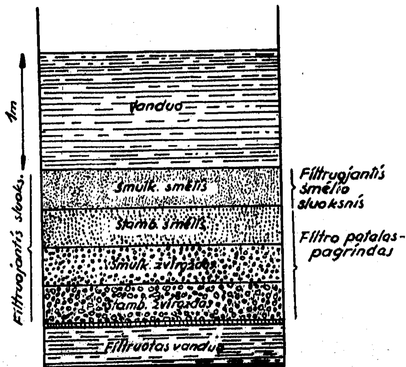
Brėž. 3. Filtrų sudėties schema
