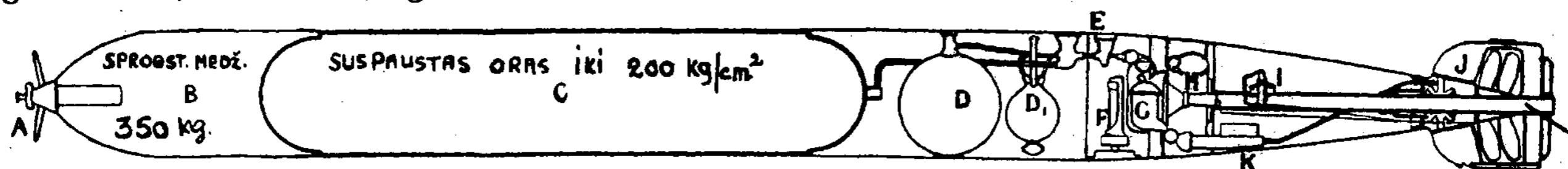
Torpedos schema: A — degtuvas ir detonatorius, B — galva su sprogstamosios medžiagos užtaisu, C — suspausto oro rezervuaras, D — vanduo, D 1 — žibalas, E — saugikliai, F — gilumos reguliatoriai, G — šildytuvas, H — mašina, I — krypties reguliatorius, J — sraigčiai ir vairai, K — tepalas
