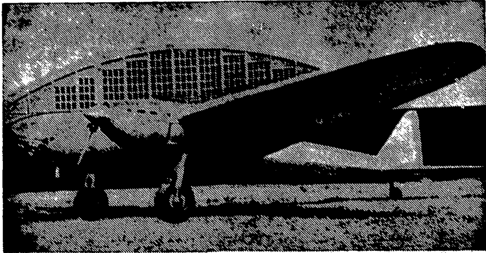
PRANCŪZIJA ATSIKOVOJO REKORDA. Prancūzų lėktuvu Amiot 370, dvimotoriu 12 Y, lakūnai mjr. Rossi ir Vigroux laimėjo 2000 km uždaros kelionės rekordą su 2000 kg krūviu, vidutinišku 437 km/val. greičiu.
