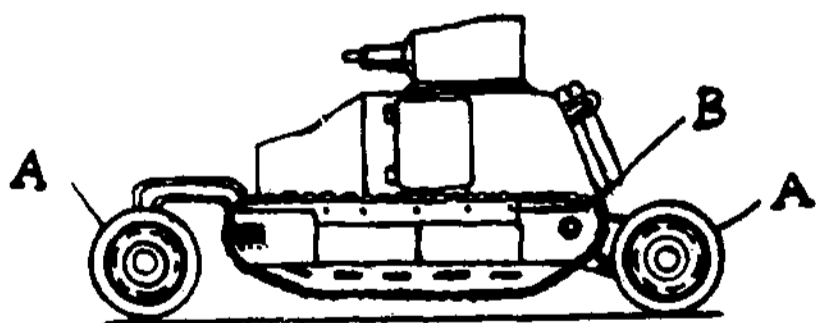
36 pieš. Universalus vikšrinis-ratinis šarvuotasis automobilis: A — ratai važiuoti keliais; B — vikšrais važiuoti be kelių.
