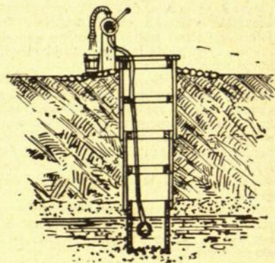
Br. 3. Lauko tipo šulinys, atviros konstrukcijos, su įleidžiama dėže be dugno ir įtaisytu rankiniu siurbliu
