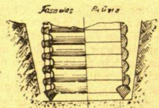
Br. 5. Šulinio rentinio nuleidimas pasikasino būdu
