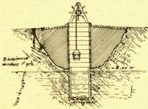
Br. 2. Lauko tipo šulinys: lentų rentinis ir vandens iškėlimo įtaisas
