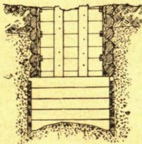
Br. 6. Rentinio nuleidimas byrančioje žemėje
