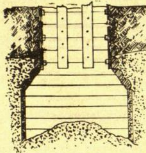
Br. 7. Rentinio sujungimas su bedugne dėže
