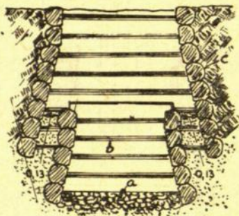
Br. 9. Rentinio pagilimas drimbantčio smėlio sluoksnyje, vandens renkamo šulinio pagalba: a) skalda, b) vandenį renkamas šulinys, c) rentinys
