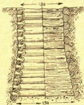
Br. 8. Rentinio nuleidimas, pereinant drimbančio smėlio sluoksnį
