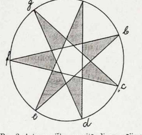
Pav. 2. Astronomiškias savaitės dienų pažėjimas. a) Mėnuolis, b) Merkuris, c) Venera, d) Saulė, e) Marsas, f) Jovis ir g) Saturnas. Šitas žvaigždės buvo žinomos senovėje ir jos sudėtos pagal senovės astronomu būdą.
