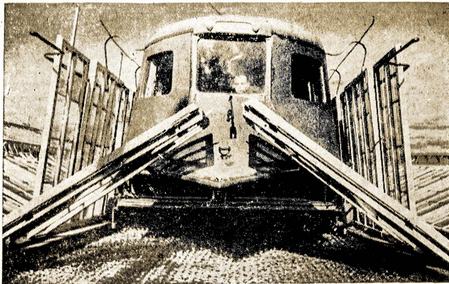
Didžiojoje Sovietų šilnamiuose varuojama tokia elektrinė mašina. Ji sudėtinga ir lygina žemę, sudaro ją į ežes, sėja, laisto, apkeipia daržoves, išravin piktžolės ir užveisia augalus sėkladulkiemis. Ši sudėtinga mašina yra sovietinis išradimas.
