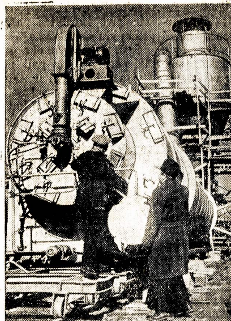
Baltijos laivų statykloje surinkti pirmieji du vitamininių žolės miltų gamybos agregatai "AVM-1,5".
