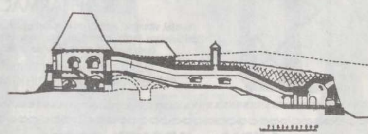
"Bokšto" kalvos artilerijos bastionas, koridorius - tunelis ir bokštas (skersinis pjūvis).
