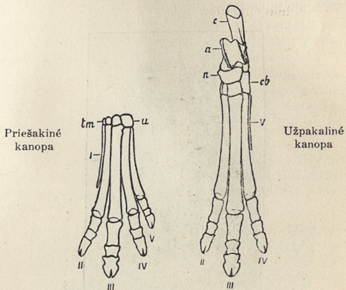
Fig. 11. Eohippo kanopa.
