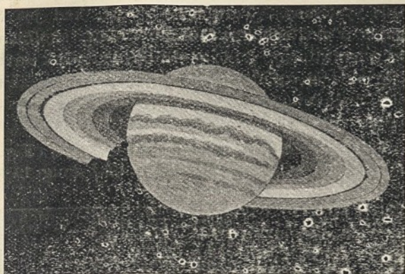
Fig. 21.— Planėta Saturnas. (Sulyg Flammariono).
