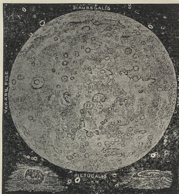
Fig. 22.— Pilnas mėnulis (pilnatis).
