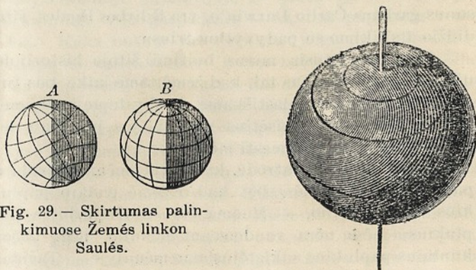
Fig. 30.-- Žemė sukasi ant savo Ašies. (Sulyg Flammariono).
