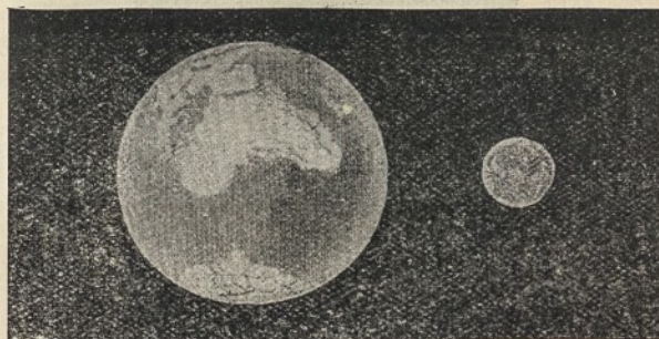
Fig. 32. — Reliatyvis didumas Žemės ir Mėnulio. (Sulyg Flammariono).
