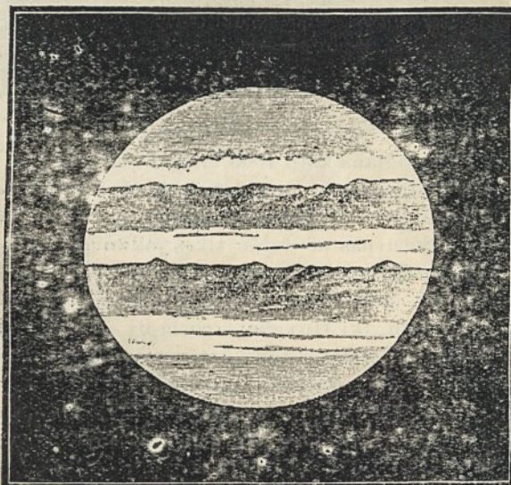
Fig. 20. — Planėta Jupiteris (sulyg Flammariono).
