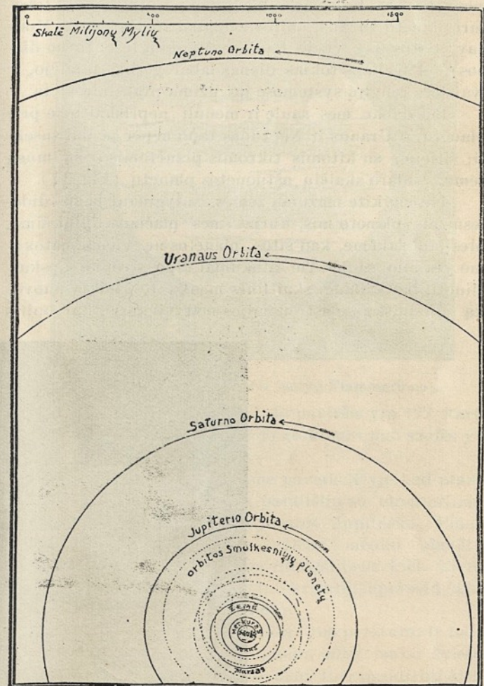
Fig. — 16. Soliarė sistema.
