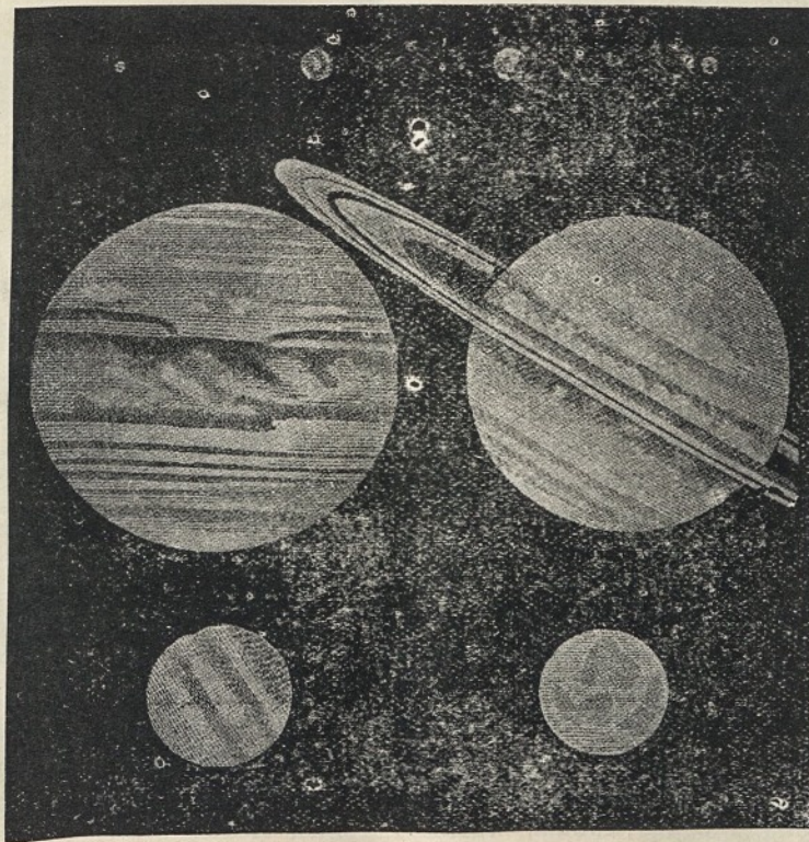
Fig. 17. - Sulygintiniai planetų didumai (sulyg Flammariono).
