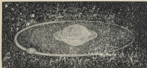
Fig. 33. — Flammarionas perstato budą, koku Žemė galėjo būti nušviesta šalin nuo saulės kaipo žiedas.
