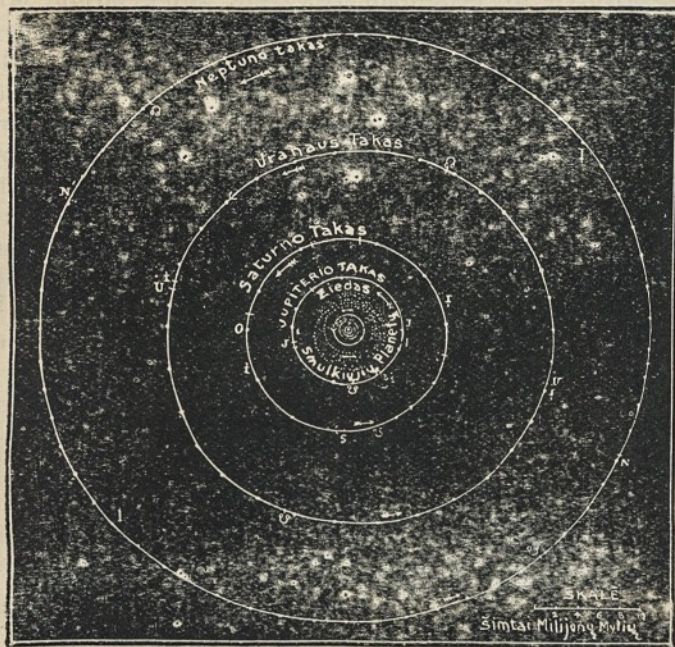
Fig. 19. — Orbitos keturiu plarėtu tilimiausiuju nuo saulės.
