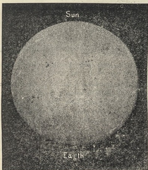
Fig. 31. — Reliatyvis diduma Žemės ir Saulės. (Sulyg Flammariono).
