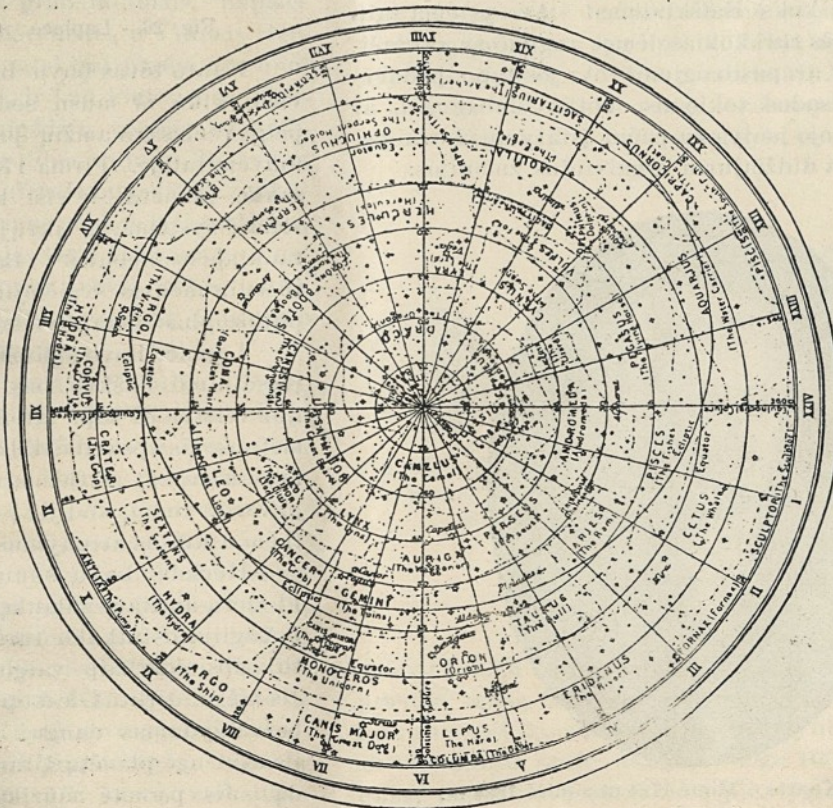
Fig. 23. — Šiaurinė žvaigždžių hémisphéra. (Sulyg Flammariono).
