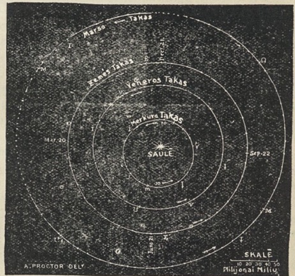
Fig. 18. — Orbitos keturiu planetų arčiausiuju prie saulės.
