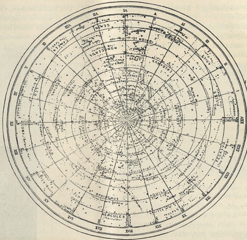
Fig. 24. — Pietinė žvaigždžių hémisphéra. (Sulyg Flammariono).
