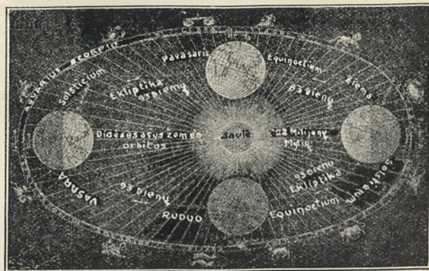
Fig. 28. Žemės orbita arba takas aplink saulę. (Sulyg Flammariono).
