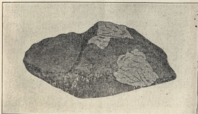
Fig. 43. — Meteoritas.
