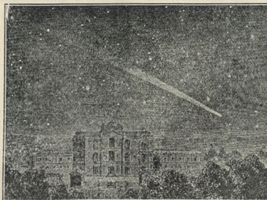
Fig. 41. — Komėta
