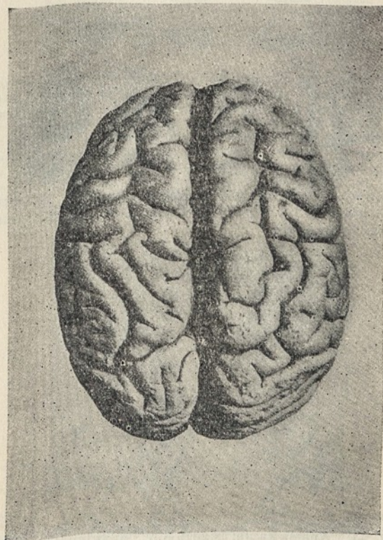
Fig. 49. Smagenis čimpanzės Sally.
