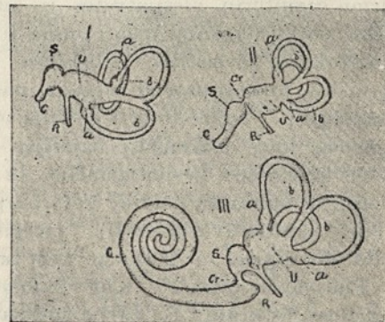
Fig. 41. Diagramos girslinio Labyrintho. I. Žuvies. II. Paukščio. III. Žindžiaus ir Žmogaus. S, sacculus; u, utriculus; c, cochlea; Cr, canalis reuniens; a, ampullae; b, pusapskričiai kanalai; R, aqueductus vestibuli.
