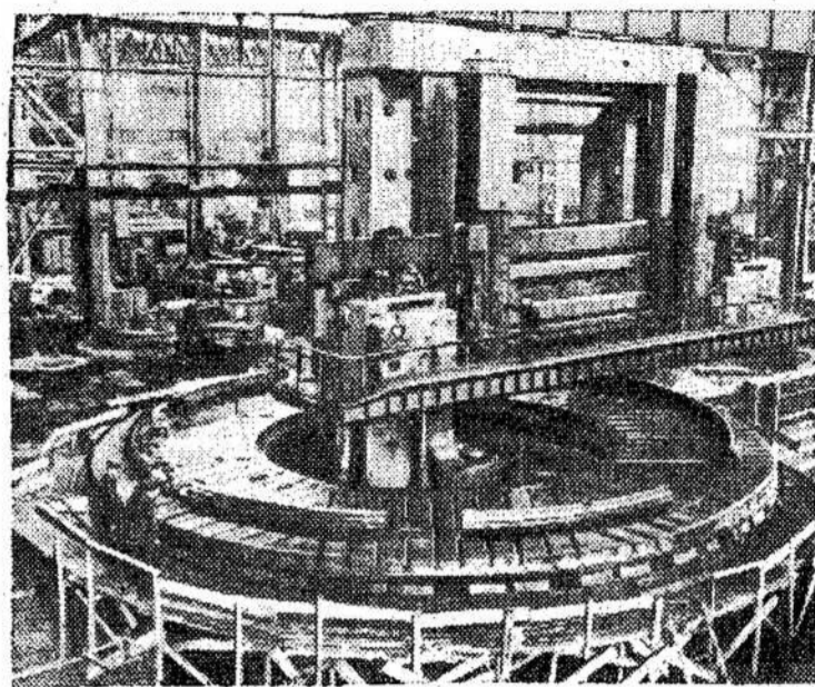
Vertikalis tekinimo įrenginys, pagamintas Tarybų Sąjungoje. Jis naudojamas gaminti turbinams grandžių. Jis sveria 260 tonų. Jo diametras 16 metrų.
