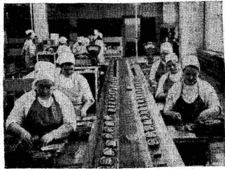
Klaipėdos žuvis apdorojimo įmonėje sumontuota pneumatinė automatizuota žuvis preservų gamybos linija. 175 gramų talpos dėžutėse gaminama silkės file ir gastronominiame užpilde ir obuolių padaže. Pradėjus jai dirbti visu pajėgumu, per parą bus patiekiami 10,000 tokių dėžūčių. (B. Aleknavičiaus nuotr.)
