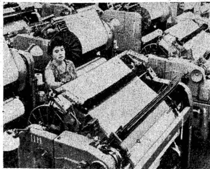
Kauno P. Ziberto šilko kombinatė nuolat atnaujinama įrengimais. Neseniai audimo ceche sumontuotos labai našios pneumatinės staklės, kurios labai paspartino darbą. (T. Žebrausko nuotrauka).
