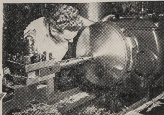
Torpedų nulyginime, elektra yra jiega užpakalyje mašinų. (Official O. W. I. Photograph.)
