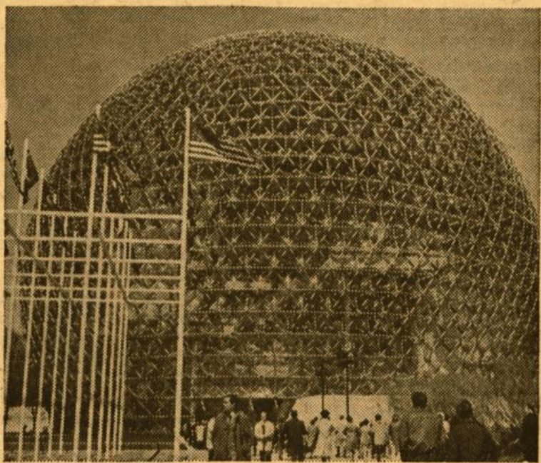
J.A.V. paviljonas pasaulinėje parodoje Expo 67 Montreaulyje. Ši paroda atžymi Kanados valstybės 100 metų sukak-tį. Didžiulį pusrutulio formos kupolą, 20 aukštų namo dydžio, suplanavo architektas R. Buckminster Fuller. Ekspонатai vėduje parodo J.A.V. atiekimus erdvų technologijoje, mene ir Amerikos istorijos momentus. 62 valstybės dalyvauja šioje 6 mėnesių parodoje, kurios tema yra "žmogus ir jo pasaulis".
