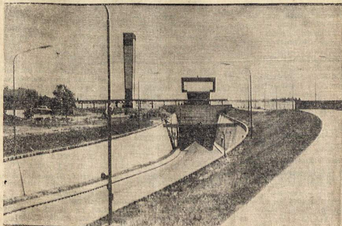
Ventiliacijos bokštas, arti 30 metrų, prie tunelio Hernandarias, trijų kilometrų ilgio, jungiančio Parana Santa Fe. Poupinio tunelio pastatymas kainavo virš trijų tūkstančių milijonų pezu.
